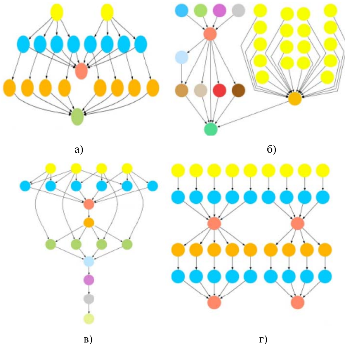
Рис. 3. Процессы: а) CyberShake; б) SIPHT; в) Montage; г) Inspiral
