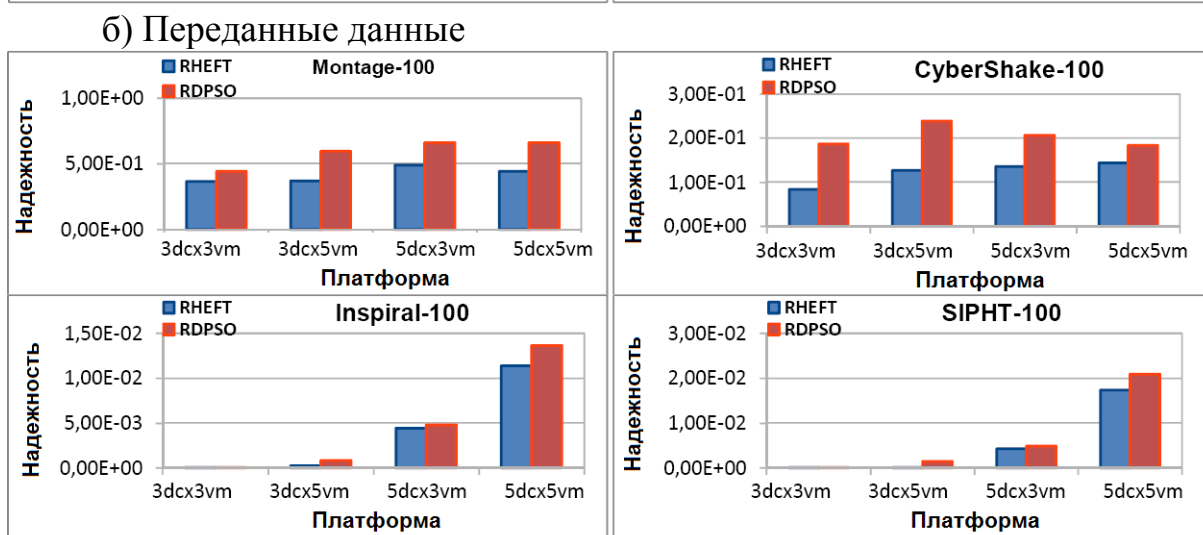
Рис. 5. а) время выполнения, б) передача данных, в) надежность на различных платформах для рабочих процессов Montage-100, CyberShake-100, Inspiral-100 и SIPHT-100
