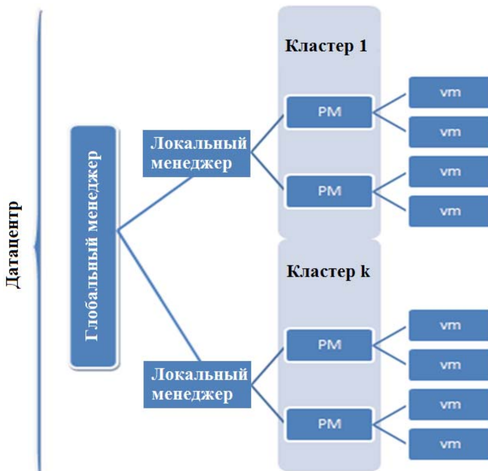
Рис. 3.10. Архитектура предлагаемой стратегии
