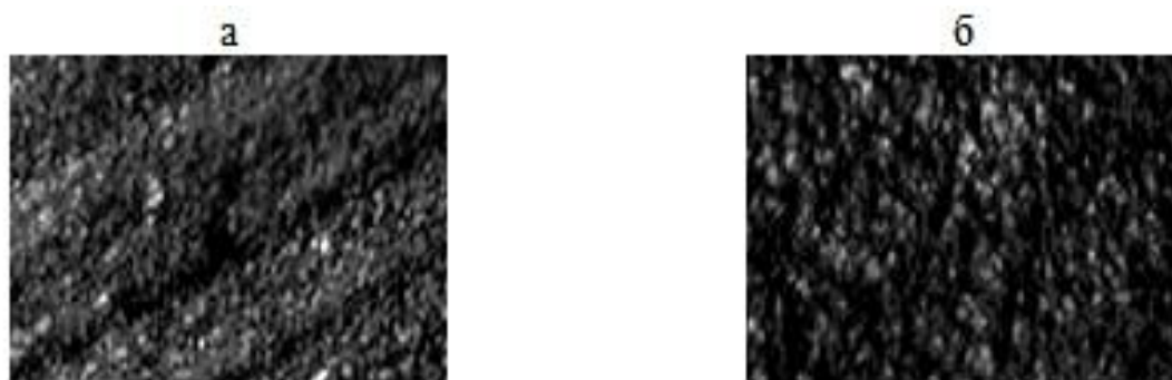
Рис. 4. Поверхность кобальтовых покрытий, полученных в режиме реверсивного тока ( \tau_k \div \tau_a = 20 \div 4 ) после отжига при 300 °С ( \times 1200 ): а – рН 1,0; б – рН 3,0
