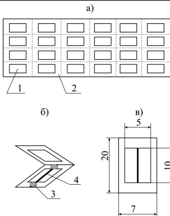
Рис. 2. Рамки для механических испытаний элементарных волокон
