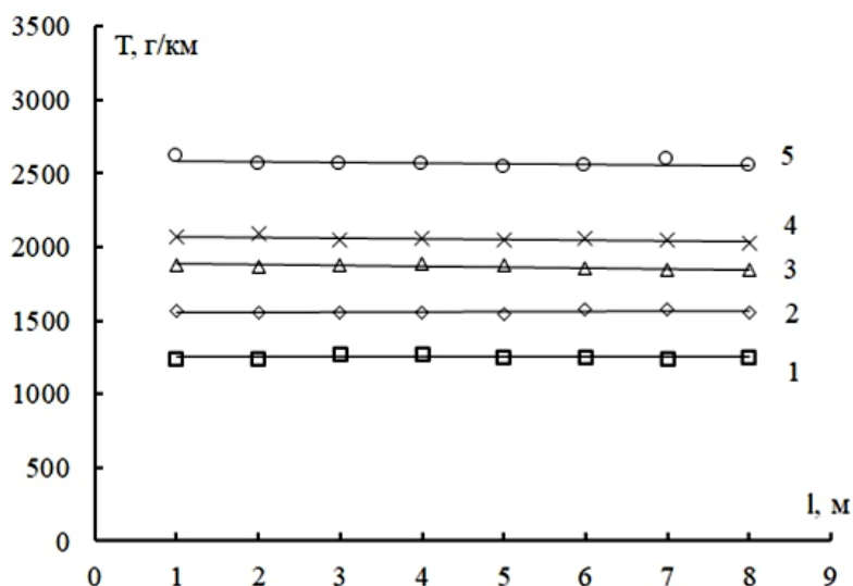
Рис. 11. Изменения линейной плотности жгутов базальтовых волокон от места замера (по длине): 1 – 1200 г/км, 2 – 1600 г/км, 3 – 1800 г/км, 4 – 2000 г/км, 5 – 2400 г/км
