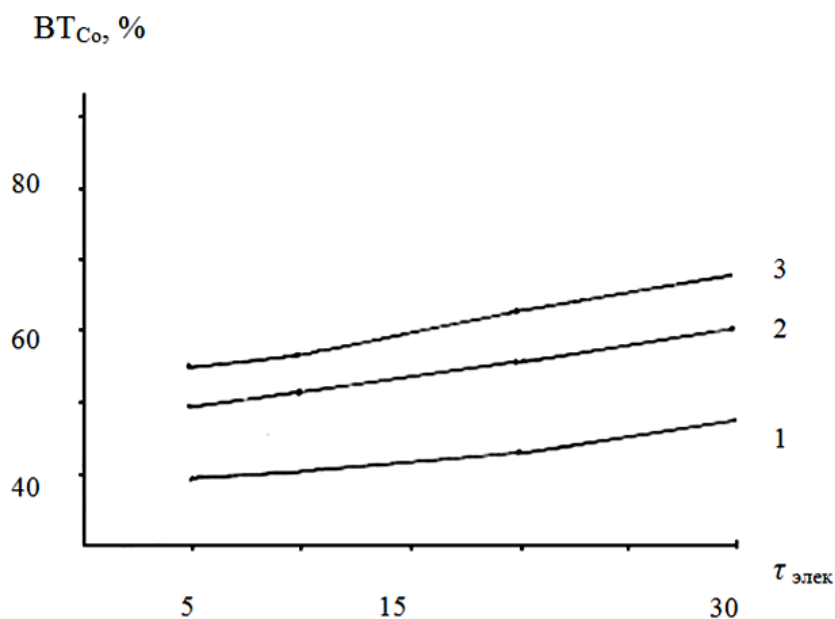
Рис. 1. Влияние катодной плотности тока ( i_k ) и продолжительности электролиза ( \tau_{\text{элек}} ) на выход по току кобальта ( \text{ВТ}_{\text{Co}} ). i_k (А/дм 2 ): 1-2; 2-4; 3-8
