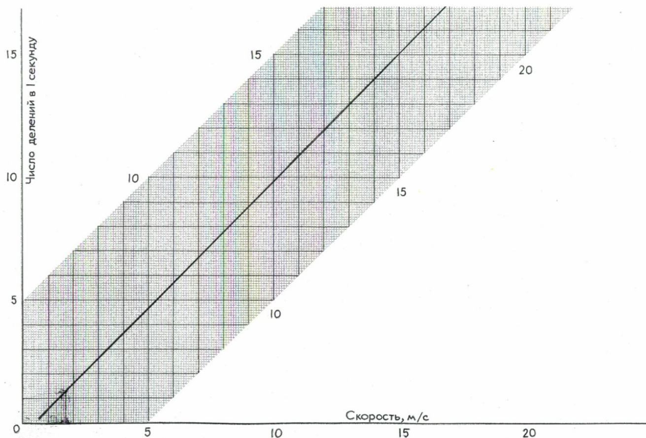
Рис. 5. Тарировочный график
