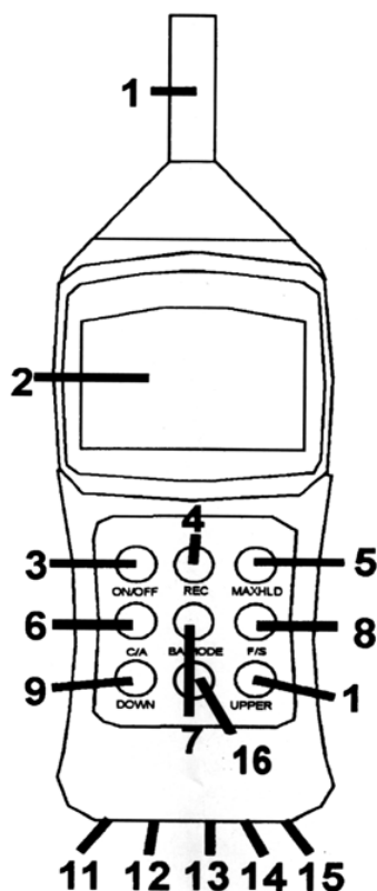
Рис. 6. Схема цифрового измерителя уровня шума:
