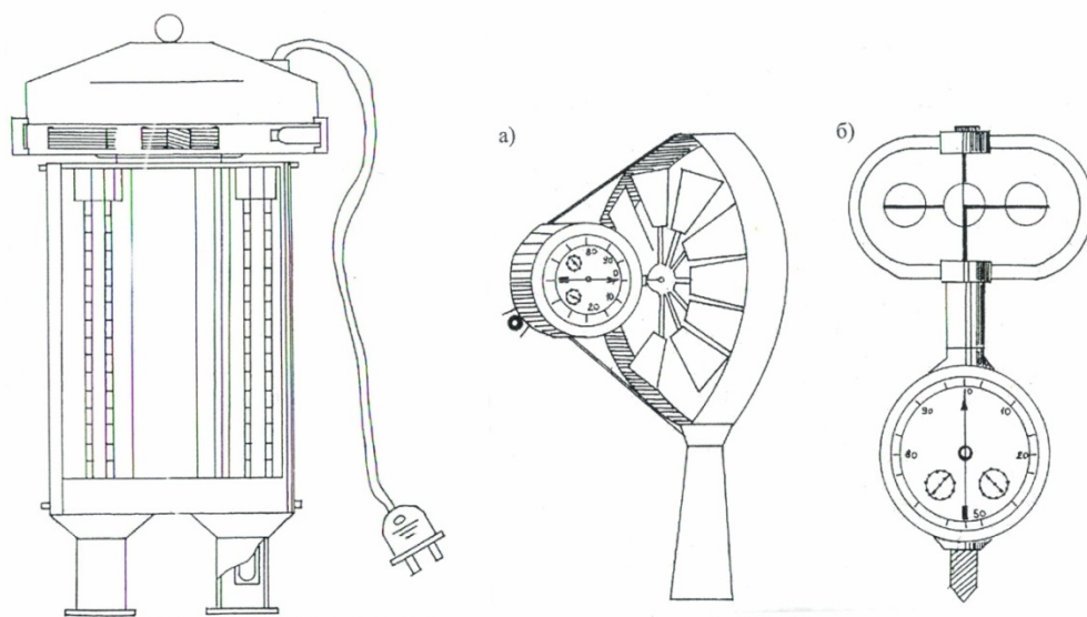
Рис. 3. Схема аспирационного психрометра и анемометров: а) крыльчатого, б) чашечного
