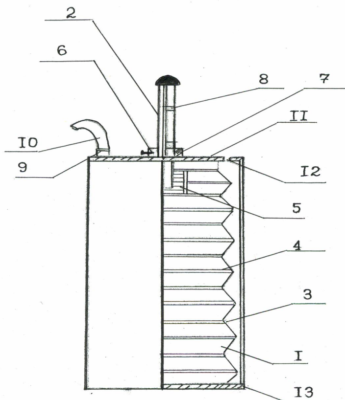
Рис. 2. Схема газоанализатора УГ-2:
