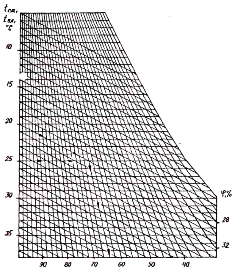
Рис. 4. Номограмма
