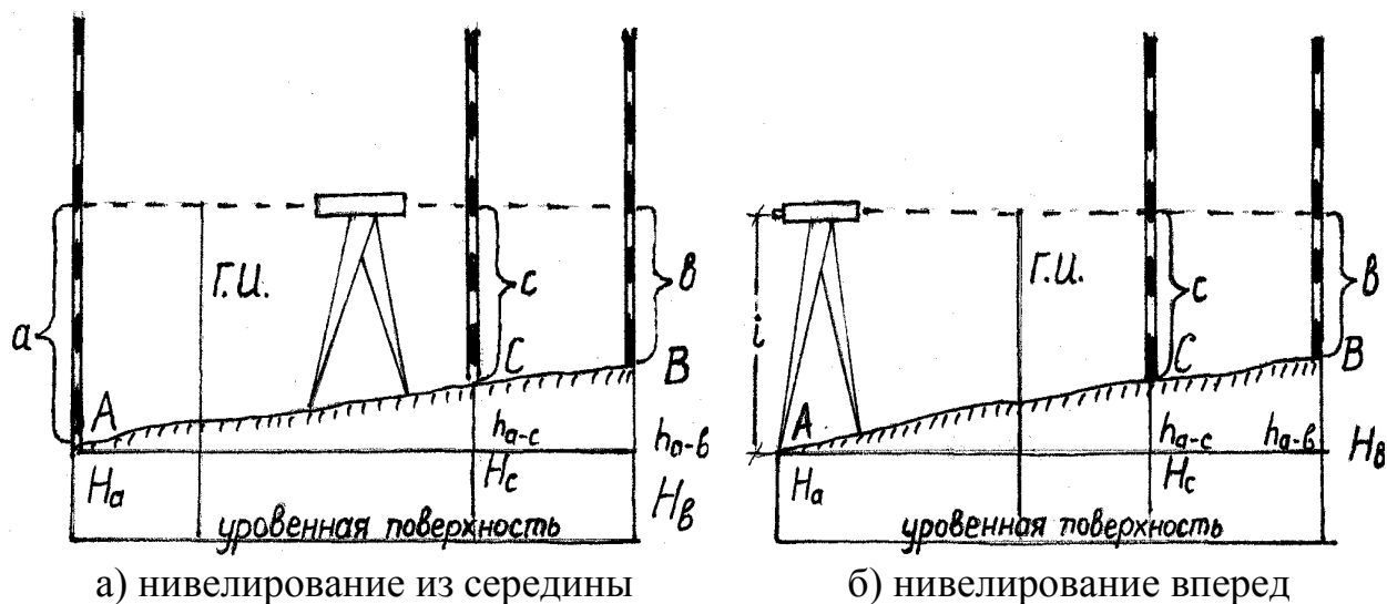
Рис. 5.6. Схемы геометрического нивелирования
