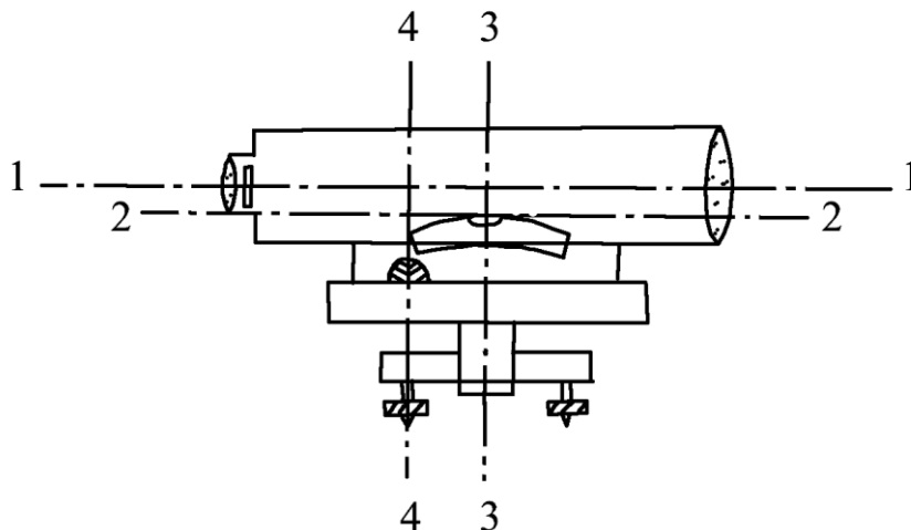
Рис. 6.1. Схема осей нивелира:
