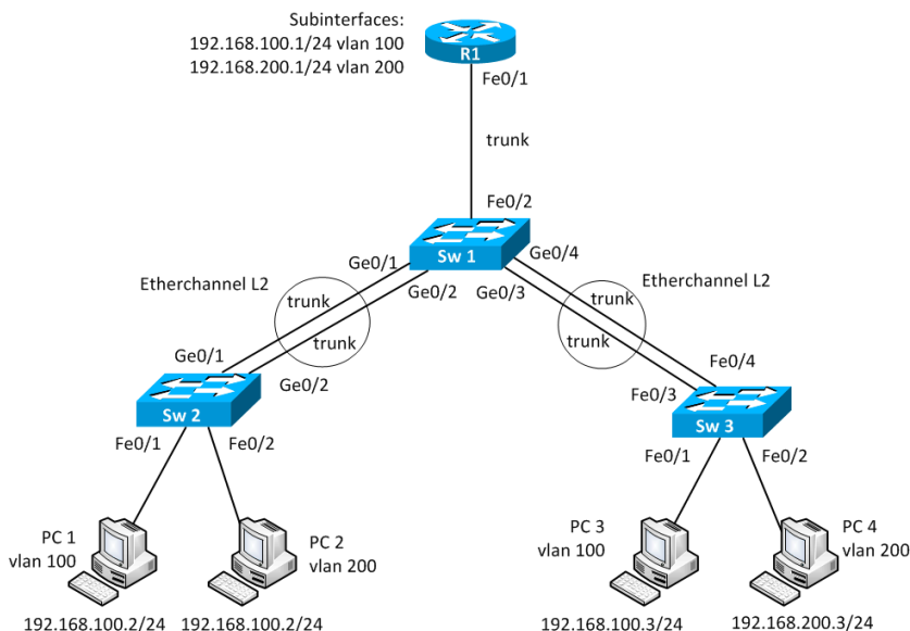
Рис. 2.9. Топология сети
