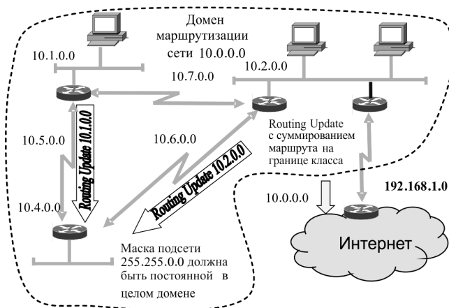
Рис. 3.7. Один домен маршрутизации
