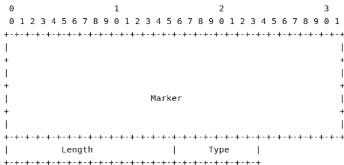
Рис. 4.4. Формат заголовка BGP-сообщения
