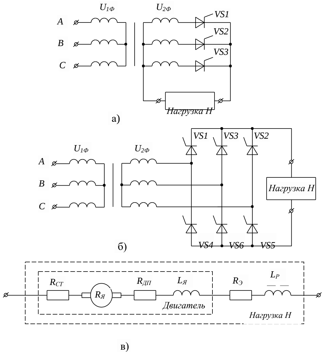
Рис. 1. Варианты схем силовых выпрямительных блоков: а – трехфазная нулевая схема; б – трехфазная мостовая схема; в – схема цепи нагрузки UB
