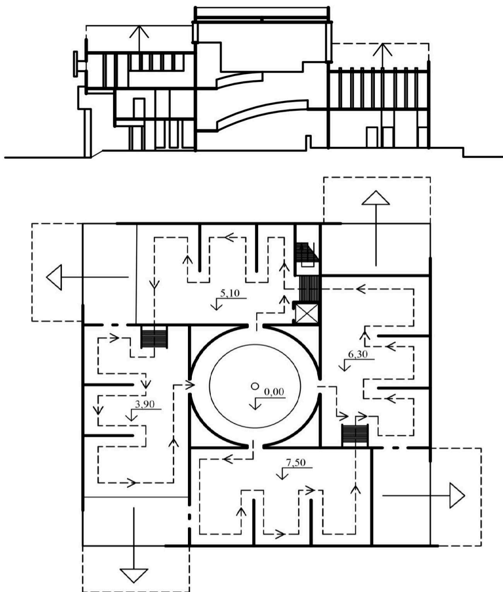
Рис. 60. Проект картинной галереи, обеспечивающий расширение здания по вертикали и горизонтали. Разрез и план здания в уровне экспозиции. Архитектор В.И. Ревякин.
