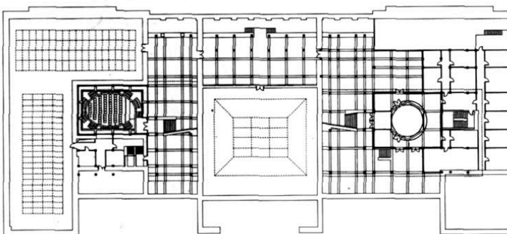
План 3-го этажа
