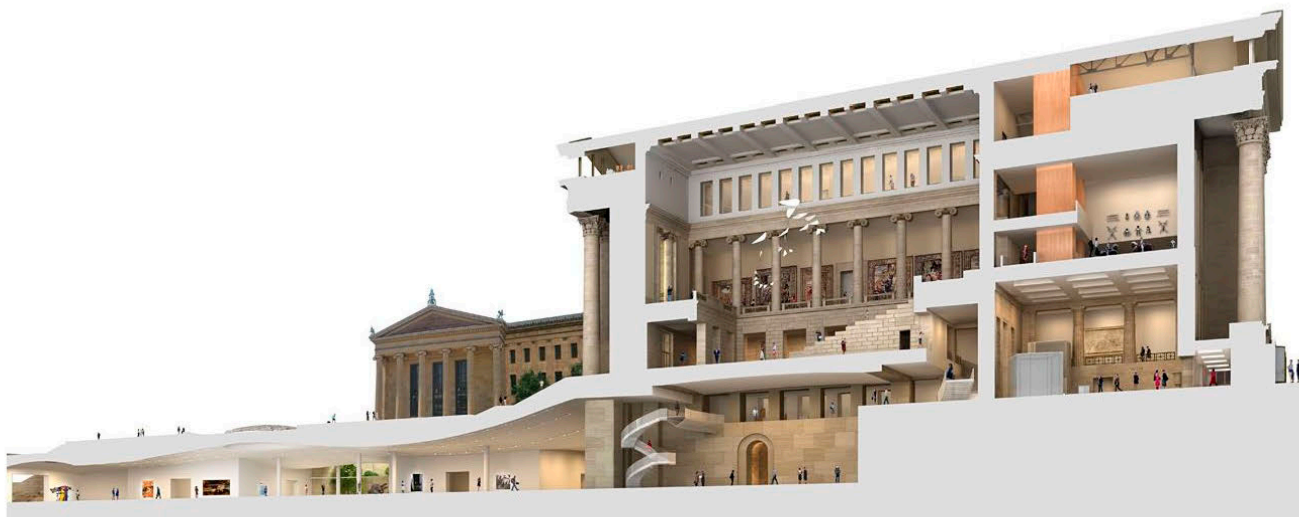
Рис. 83. Музей искусств в Филадельфии, США [53]. Проект реконструкции. Разрез. Архитектор Френк Гери
