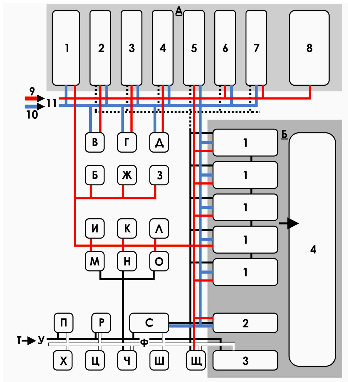
Рис. 66. Состав и взаимосвязь помещений художественного музея (по В.И. Ре- вякину): А – фондохранилище; 1. – приемная экспонатов с изолятором; 2 – рабочее помеще- ние с каталогами, фототекой и научным архивом; 3 – хранилище живописи; 4 – хранилище скульптуры; 5 – хранилище графики; 6 – хранилище прикладного искусства; 7 – сейфовое хра- нение; 8 – техническое помещение; 9 – график движения сотрудников; 10 – путь переме- щения экспонатов; 11 – служебный вход; Б – экспозиционная часть; 1 – постоянная экспо- зиция; 2 – зал временных выставок; 3 – зона отдыха; 4 – открытые экспозиционные площади; В – дезинфекционная камера; 7 – фотолаборатория; Д – реставрационные мастерские; Е – склад музейного оборудования; Ж – слесарная мастерская; З – столярная мастерская; И – кабинеты научных работников; К – комнаты персонала; Л – санитарные блоки; М – библио- тека; Н – администрация; О – помещения для занятия кружков; Я – касса; Р – киоск; С – лек- ционный зал; Г – график движения посетителей; У – главный вход; Ф – контроль; Х – пост охраны; Ц – гардероб; Ч – экскурсионное бюро.
