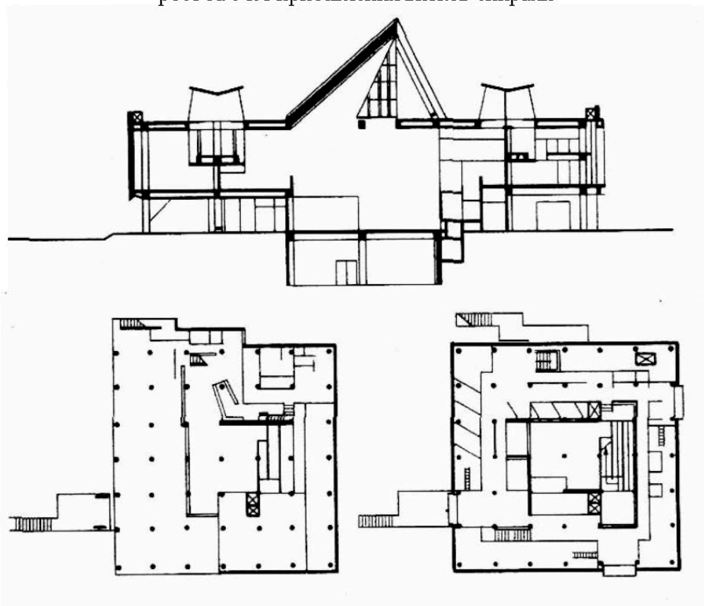
Рис. 27. Национальный музей западного искусства в Токио. Разрез, план 1 этажа, план 2 этажа. Архитектор Ле Корбюзье
