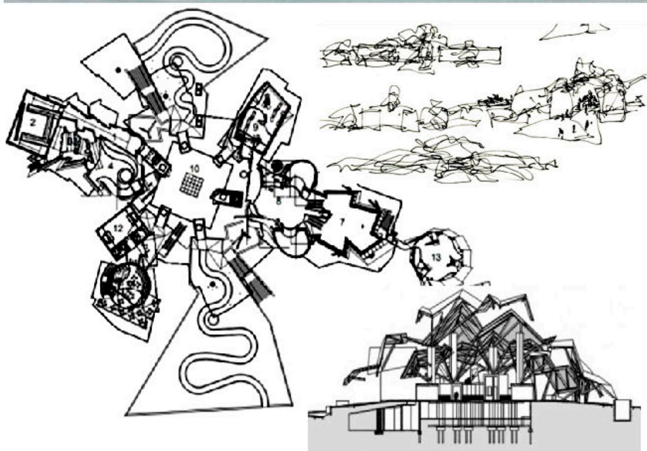
Рис. 62. Biomuseo – музей биоразнообразия, Панама, 2014 год. Панорама города, серия эскизов, план и разрез музея [48]. Архитектор Френк Гери
