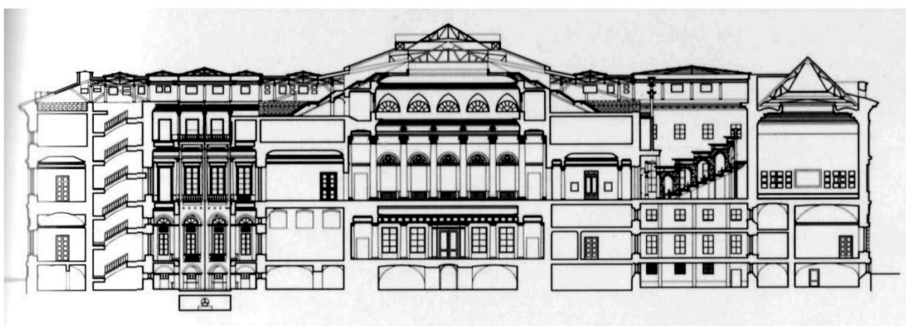
Рис. 92. Продольный разрез дворца
