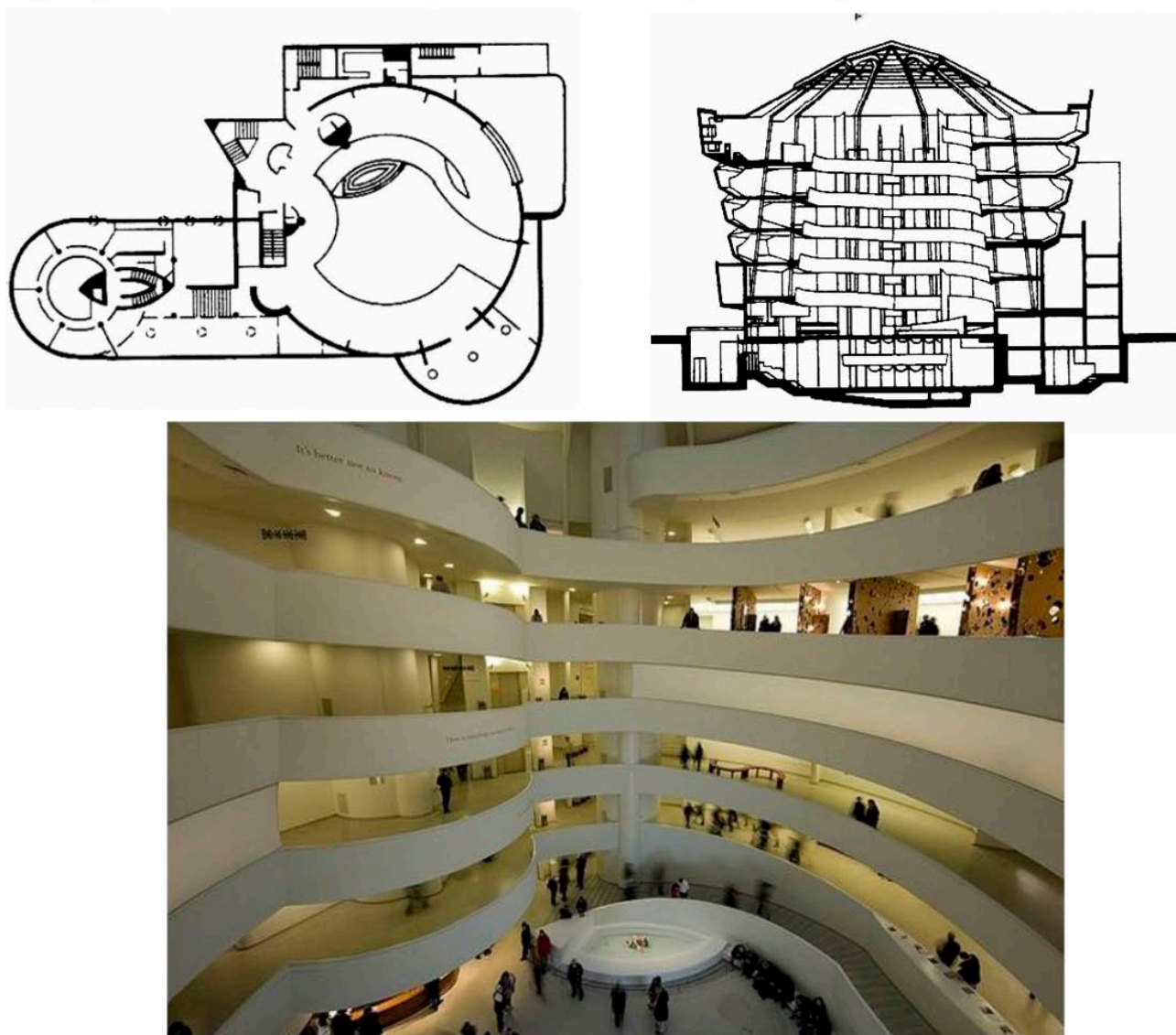
Рис. 24. Музей Соломона Гугенхайма, Нью-Йорк, США, 1959 год. План, разрез, интерьер. Архитектор Фрэнк Ллойд Райт
