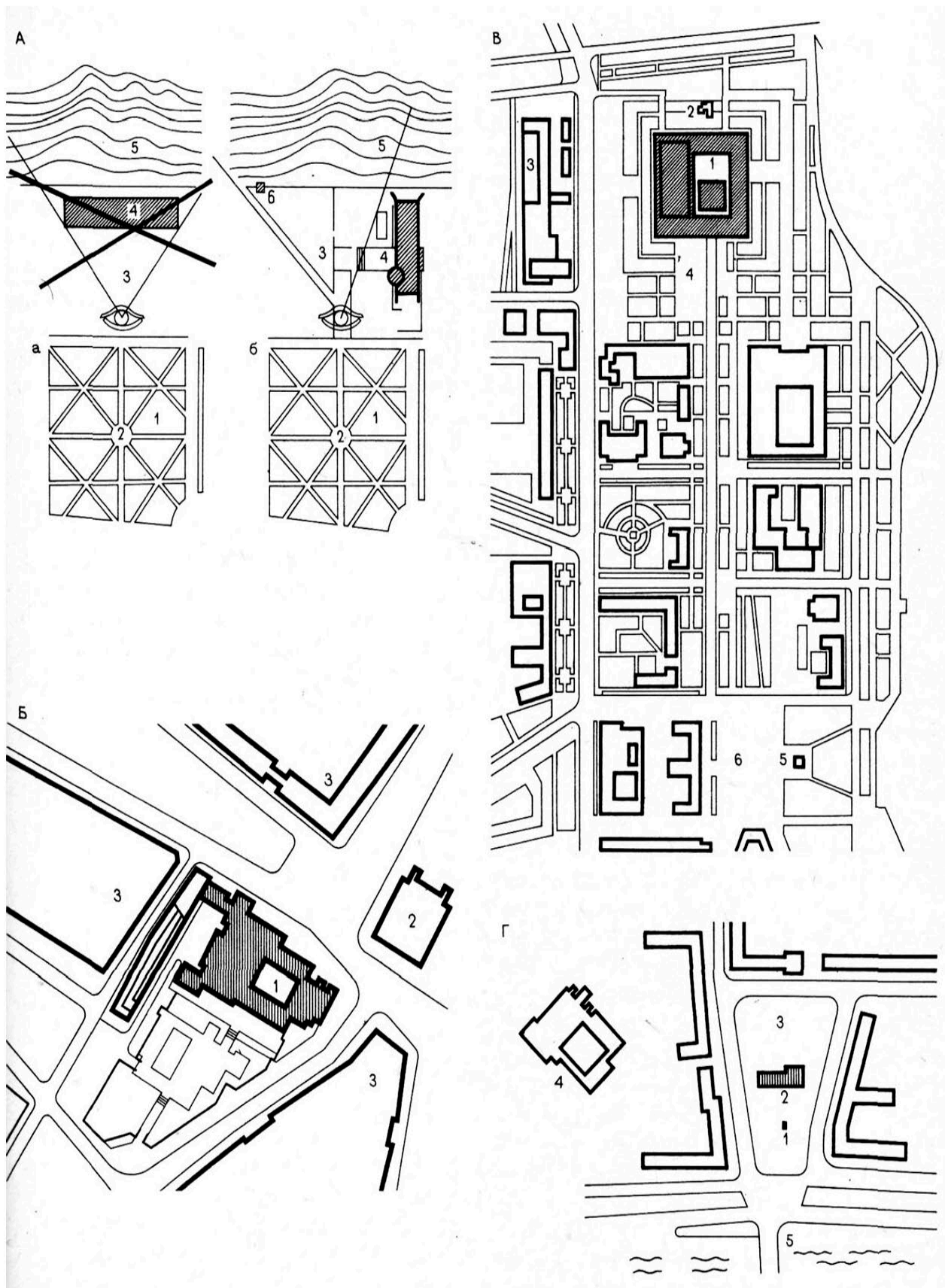
Рис. 61. Примеры расположения музейного здания в архитектурно-планировочной структуре города [3, с. 263]
