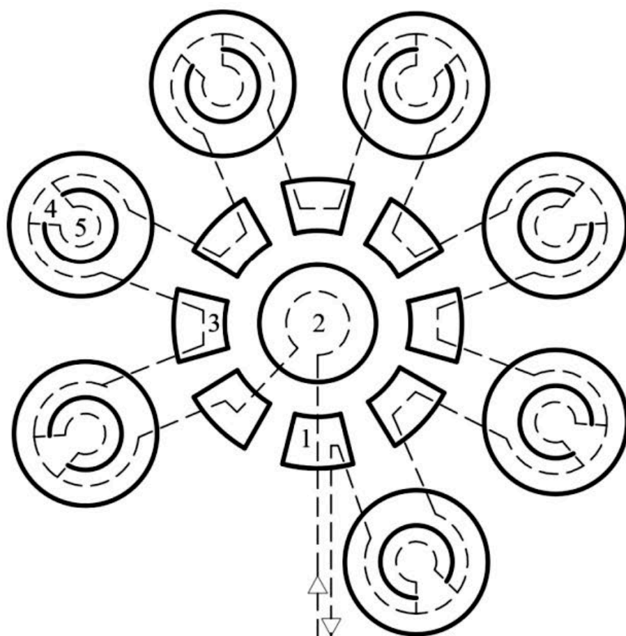
Рис. 67. Принципиальная схема движения (по Ф. Мицисси):
