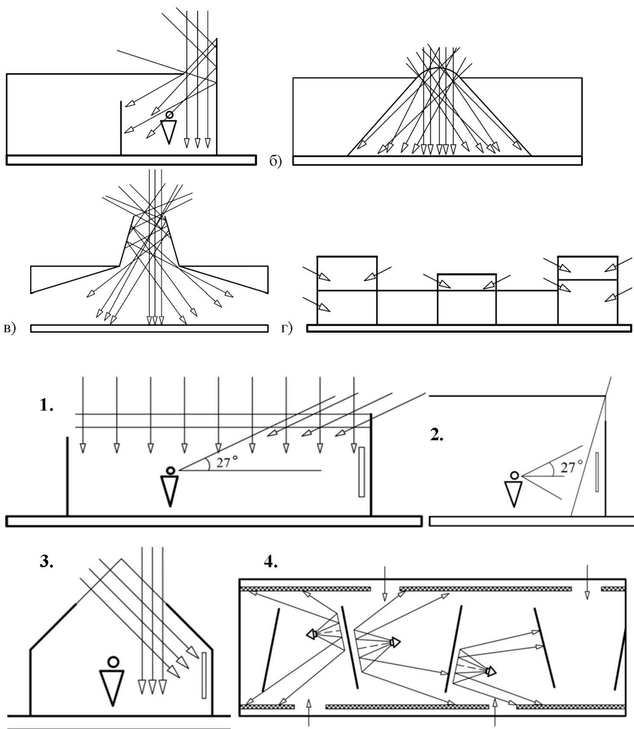
Рис. 74. Схемы освещения экспозиции (по В.И. Ревякину):
