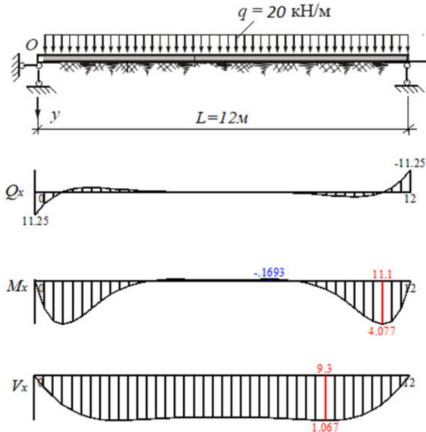
Рис.8.1 Эпюры V_x, M_x, Q_x
