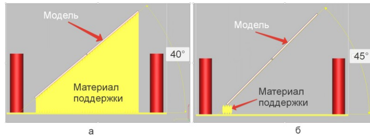
Рис. 17. Моделирование материала поддержки при угле наклона менее 45 градусов (а) и равным 45 градусов (б)
