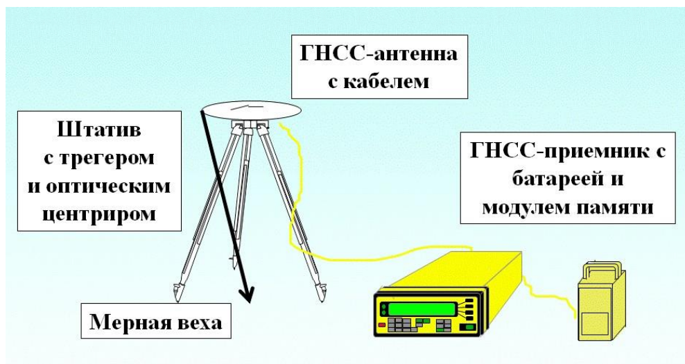
Рис. 9. Состав комплекта ГНСС оборудования для проведения статических измерений
