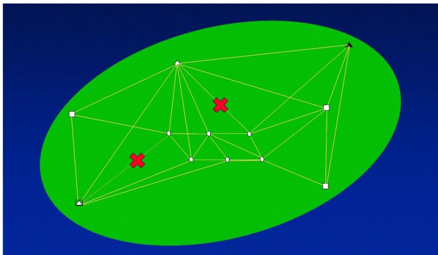
Рис. 13 Пример свободной сети с одной исходной точкой
