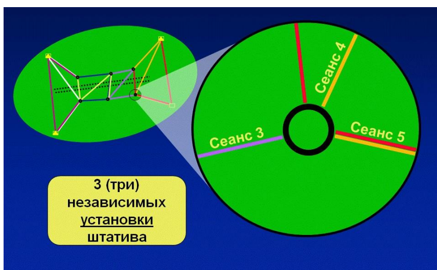
Рис. 7. Пример пунктов с несколькими независимыми сеансами измерений
