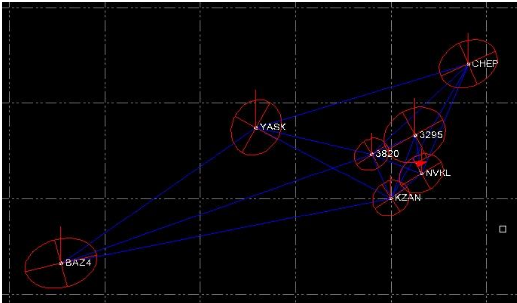
Рис. 14 Пример уравнивания свободной сети
