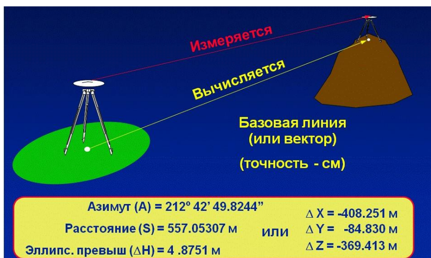
Рис. 12 Измеряемые и вычисляемые параметры базовых линий
