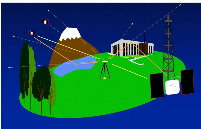
Рис. 8. Препятствия и источники многолучевости (многопутности) при проведении ГНСС измерений
