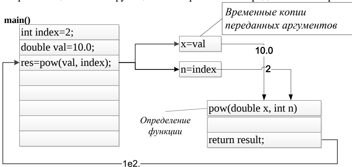
Рису.9.3. Передача параметров по значению
