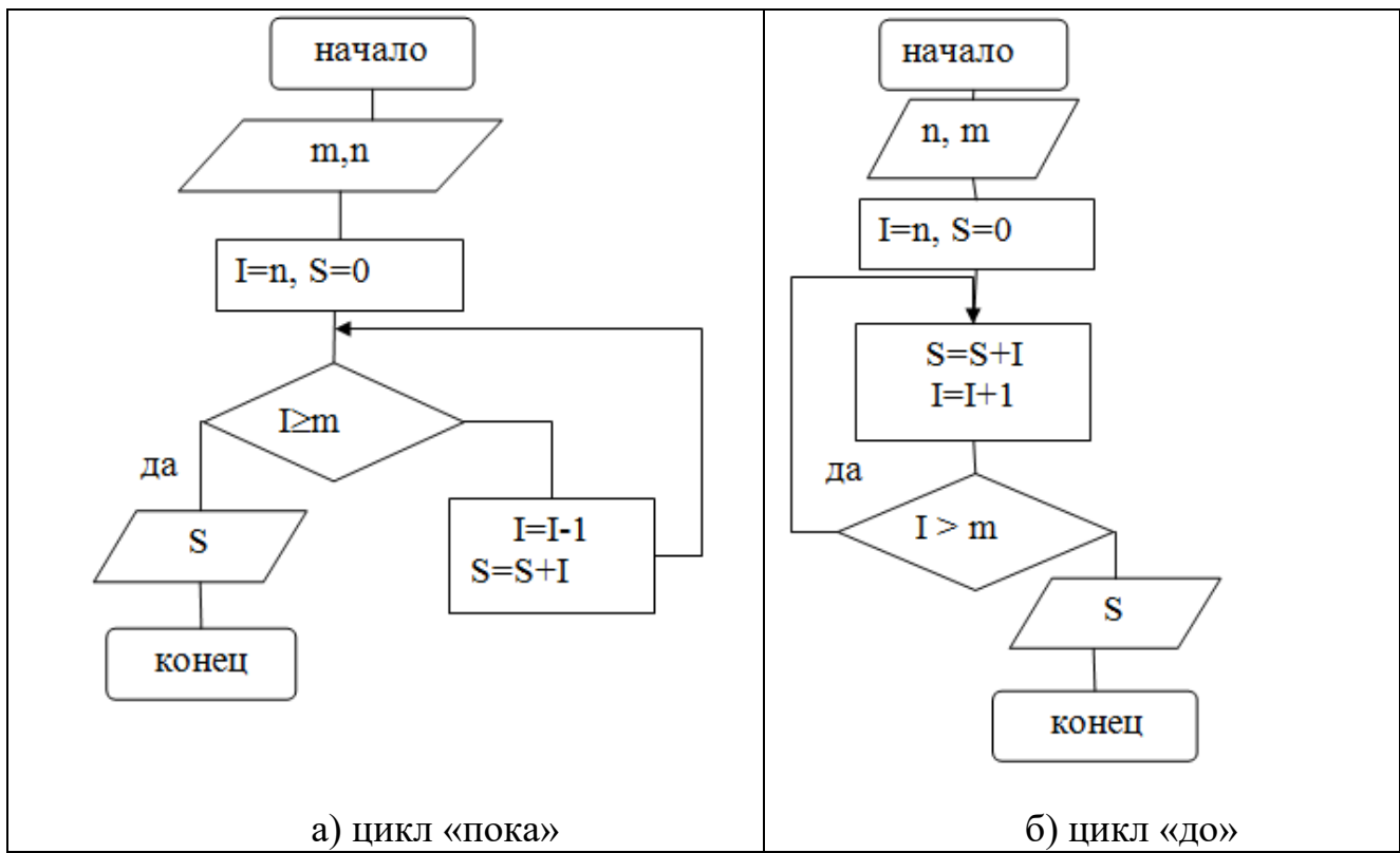
Рис. 7.3. Блок-схема алгоритма вычисления суммы последовательных чисел
