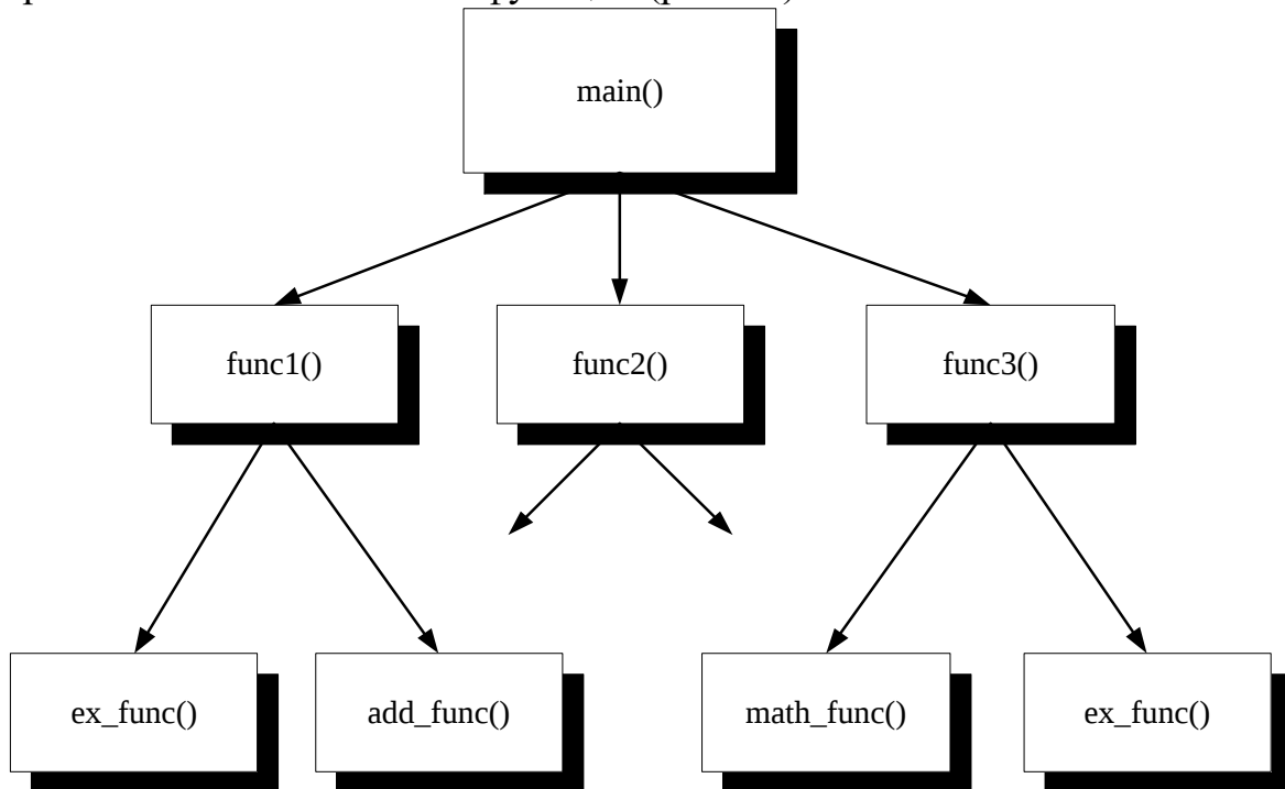
Рис. 9.1. Иерархия функций в программе на Си
