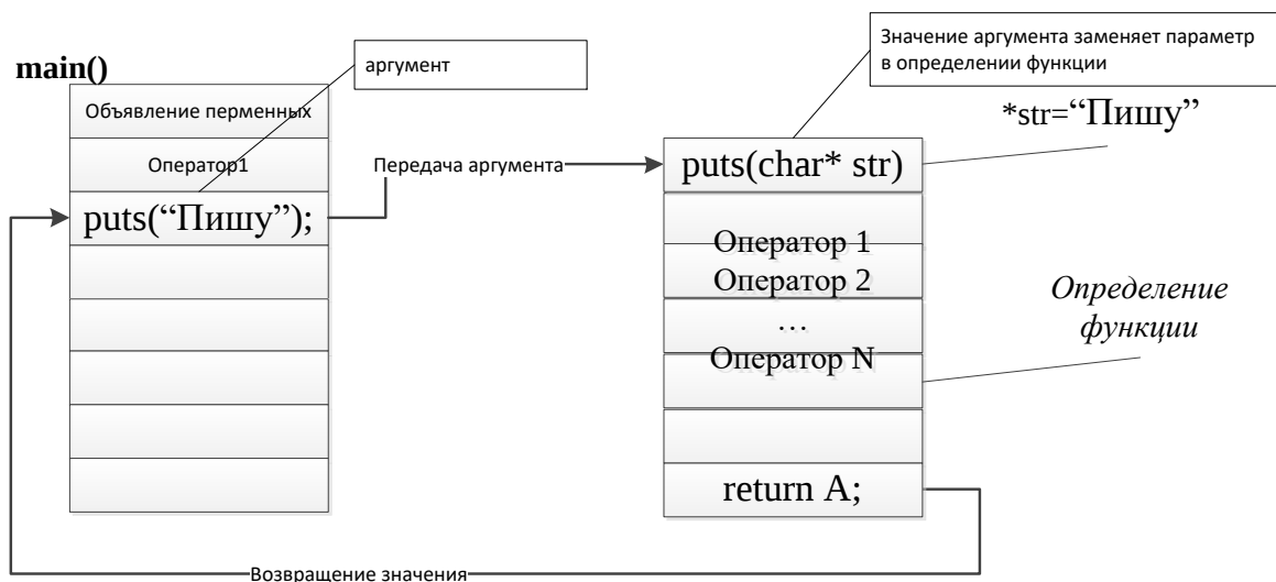
Рис.9.2. Организация программы с использованием функций
