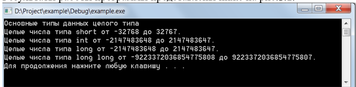
Рис.3.1. Результат работы программы
