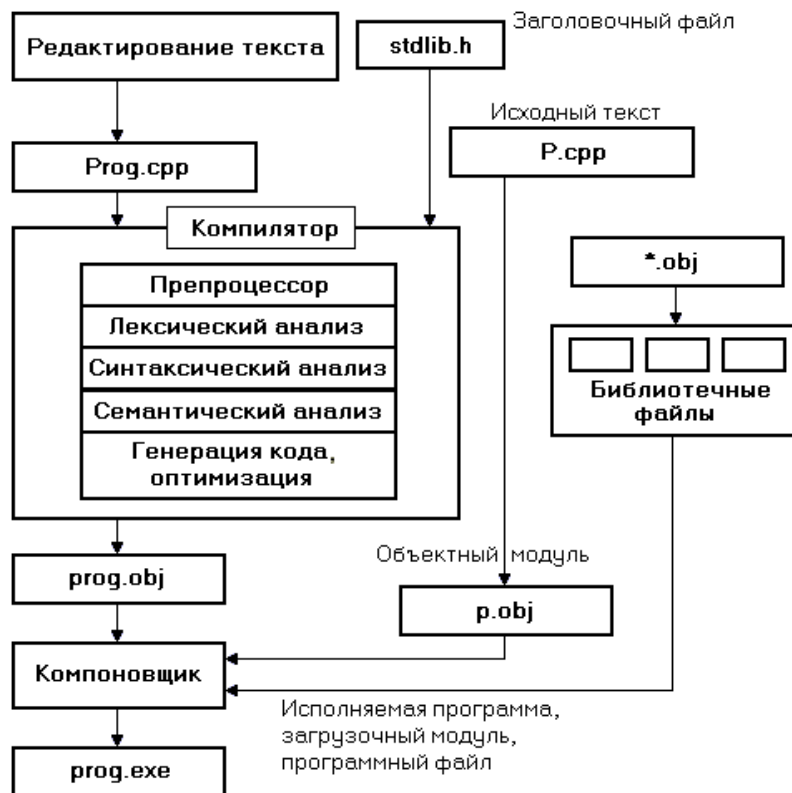
Рис. 1.1. Процесс создания программы
