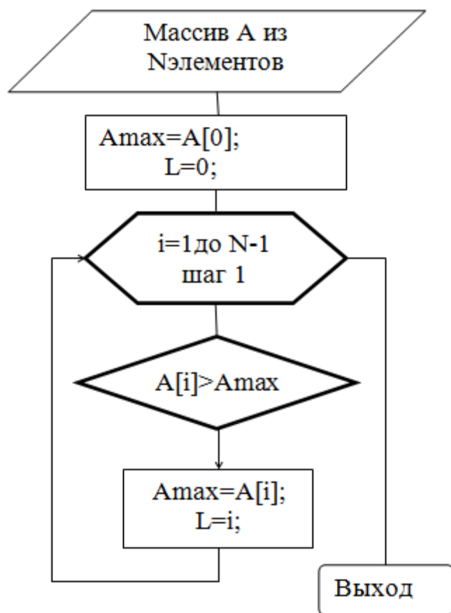
Рис. 15.2. Алгоритм линейного поиска
