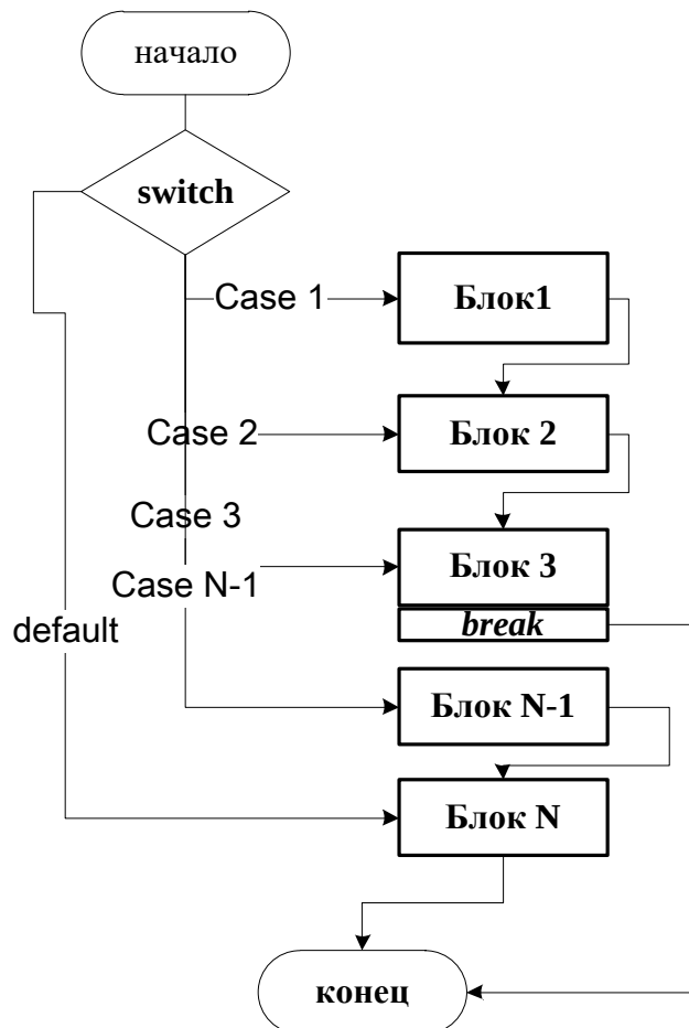
Рис. 6.1. Управление ветвлением с операторами switch и break
