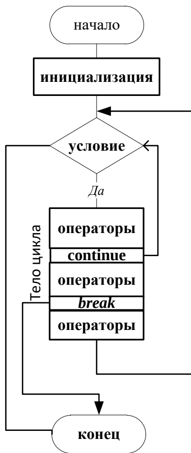
Рис. 7.2. Управление циклом с операторами break и continue
