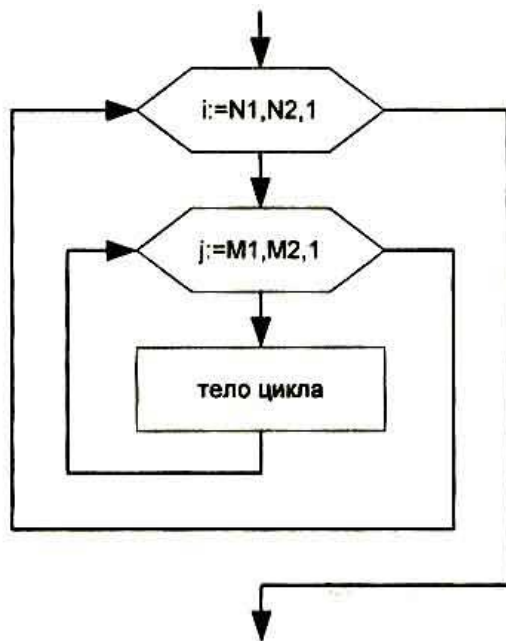
Рисунок 8.1. Блок-схема алгоритма с внутренним циклом
