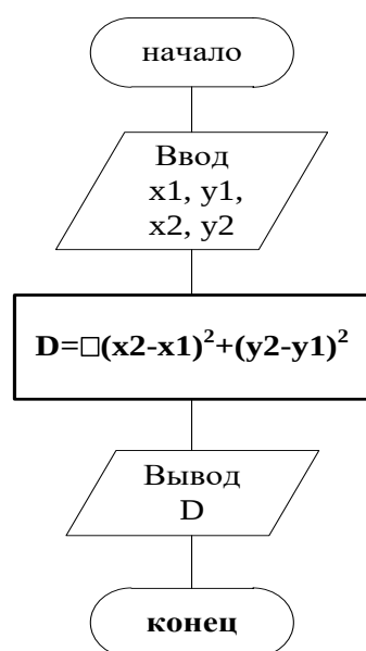
Рис. 4.3. Блок-схема алгоритма
