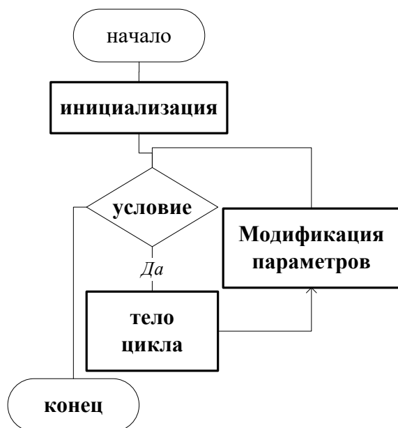
Рис.7.1. Цикл
