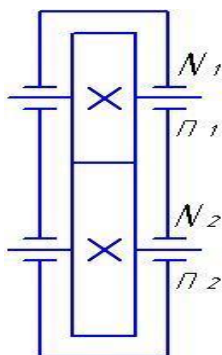
Рис. 6 Схема редуктора
