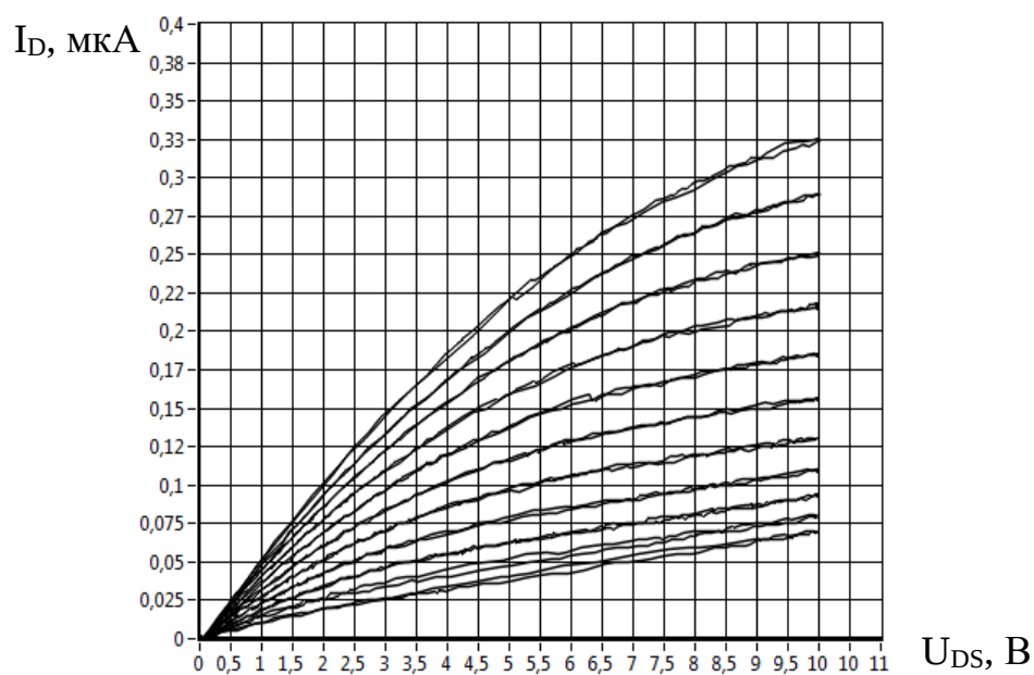
Рисунок А.2 – ВАХ TTFT, измеренная на лабораторном стенде
