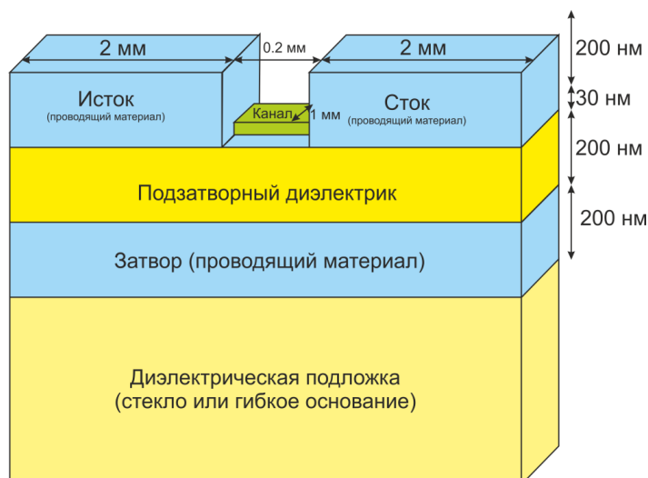
Рисунок А.1 – Схема прозрачного тонкопленочного металлооксидного транзистора
