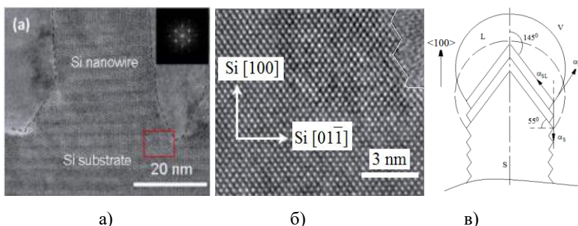
Рис. 16. ПЭМ-изображение ННК Si, выросшего в направлении \langle 100 \rangle на Si-подложке (100) (а), увеличенное изображение участка этого кристалла (б) [164] и схема выращивания ННК в направлении \langle 100 \rangle (в)
