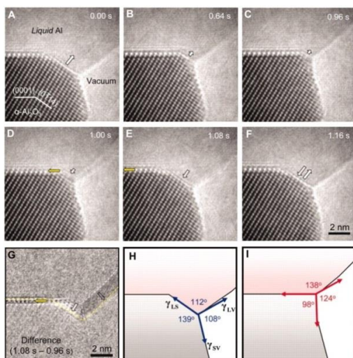
Рис. 30. Покадровая видеосъемка в ПЭМ окрестности ТЛ НКК \alpha\text{-Al}_2\text{O}_3 , иллюстрирующая изменение площади усечения (А-Г) и схема треугольника сил, соответствующих свободной поверхностной энергии границ раздела фаз (Н, I) [117]
