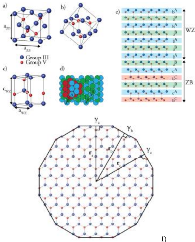
Рис. 32. Элементарная ячейка ZB полупроводникового соединения в различных ориентациях (а, б). Элементарная ячейка WZ (с). Плотнупакованные слои: кубическая упаковка слева и гексагональная упаковка справа (д). ZB и WZ ячейки в одной и той же структуре, демонстрирующие плотнупакованные последовательности укладки (е). Двумерный кристалл с равновесной кристаллической формой, которую можно описать теоремой Вульфа (ф) [234]
