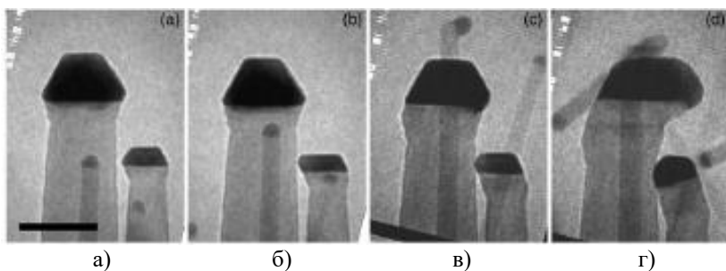
Рис. 13. Серия светлопольных изображений, полученных при выращивании in situ кремниевых ННК из дисилана с использованием наночастиц сплава AuAl: а) ННК в процессе роста при 575 °С; б) Те же ННК через 81 с роста; в) через 290 с роста; г) ННК в процессе роста при 495 °С через 500 с. Темная линия – граница двойника, образовавшегося при изменении температуры. Масштабная линейка 25 нм [151]
