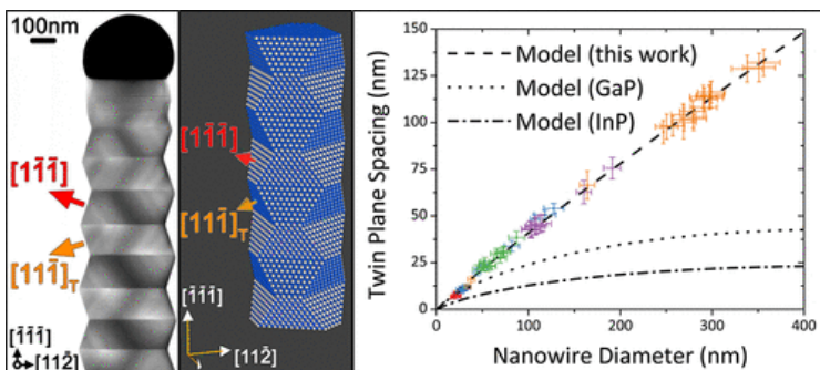
Рис. 26. Периодическое расположение двойниковых плоскостей сверхрешеточной структуры ННК GaAs (слева) и линейная зависимость расстояния между плоскостями двойникования и диаметром ННК (справа) [209]
