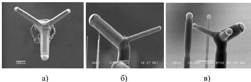
Рис. 19. Неуправляемый ПЖК-рост ННК \text{Si}_x\text{Ge}_{1-x} , приводящий к разрыву капли и ветвлению кристалла (а–в)
