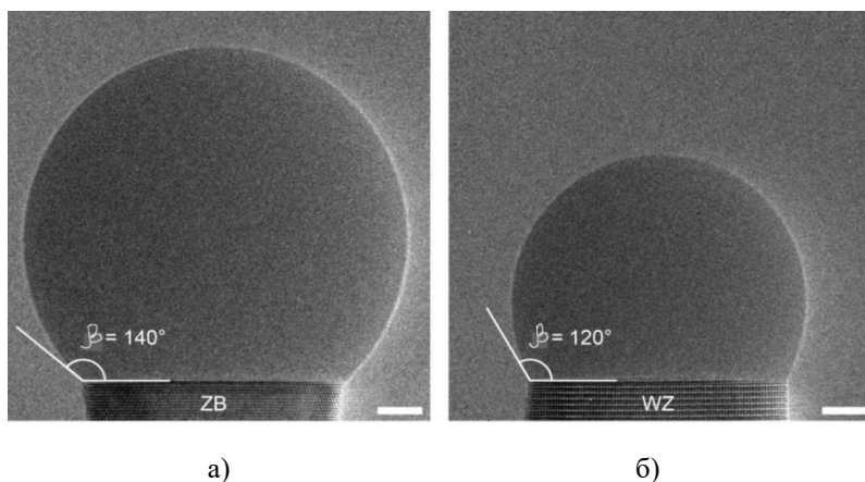
Рис. 8. Изображения вершин ННК GaAs со структурами ZB (а) и WZ (б) [91]. Катализатор – Ga
