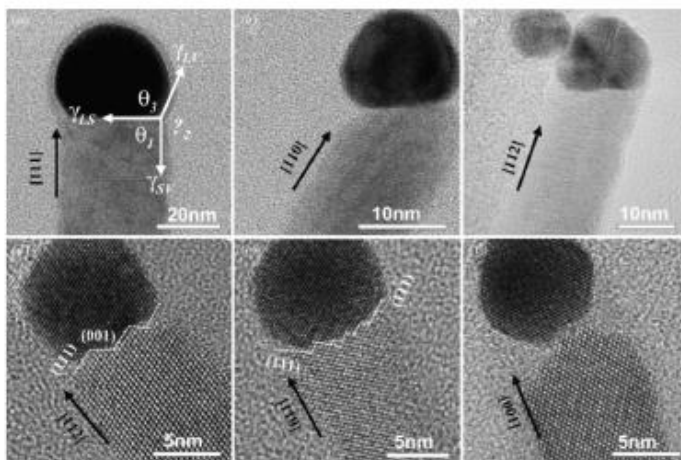
Рис. 18. ТЕМ-изображения ННК ZnSe, выращенных вдоль направлений (a) \langle 111 \rangle , (b) и (e) \langle 110 \rangle , (c) и (d) \langle 112 \rangle и (f) \langle 001 \rangle . В целом Взаимосвязь между нанопроводом Au и ZnSe представляет собой либо одну (111) поверхность (a) - (c), либо комбинацию самой низкой энергии (111) и (001) поверхностей (d) - (f) [165]
