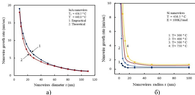
Рис. 10. Экспериментальная (1) и теоретическая (2) зависимости скорости роста ННК InAs от радиуса (температура роста T=440^\circ\text{C} ) [144] (а) и теоретические зависимости (1-4) скорости роста ННК Si от радиуса [143] (б)
