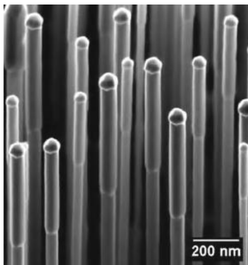
Рис. 33. Гетероструктурные ННК InAs-InSb [239]
