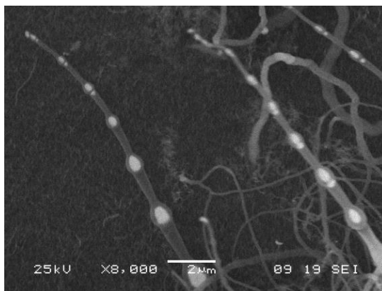
Рис. 6. Радиальная периодическая неустойчивость роста ННК Ge в системе Au-Ge с периодическим захватом катализатора
