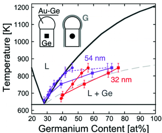
Рис. 21. Фазовая диаграмма Au–Ge, иллюстрирующая изменение предельной концентрации Ge при равновесии в крупных (макроскопических) и малых (наноскопических) каплях металлического катализатора [185]
