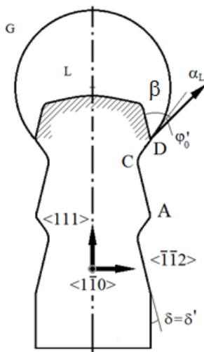
Рис. 37. Схема фасетирования боковой поверхности ННК по ПЖК-механизму
