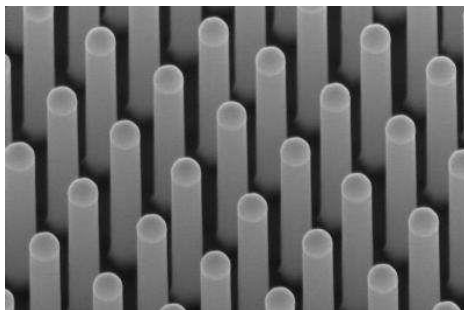
Рис. 1. РЭМ-изображение регулярной системы цилиндрических ННК InP диаметром 180 нм и длиной 1.5 мкм, выращенных по ПЖК-механизму. Катализатор – Au [28]
