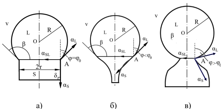
Рис. 15. Схема сопряжения границ раздела фаз пар, жидкость, кристалл на ТЛ при 0 < \varphi < 90^\circ и R = \text{const} (а), увеличении R (б), уменьшении R (в). Здесь \delta – угол наклона боковой поверхности ННК
