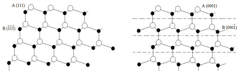
Рис. 25. Преобразование структуры цинковой обманки (слева) в структуру вюрцита (справа). Пунктирными линиями обозначены плоскости двойникования. Плоскости цинковой обманки A\{111\} и B\{111\} сравнимы с плоскостями A\{0001\} и B\{0001\} вюрцита
