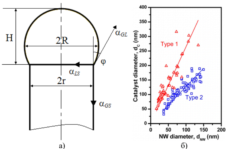
Рис. 12. Схема капли катализатора на вершине ННК (а) и соотношение диаметра капли катализатора и диаметра ННК, иллюстрирующее постоянство угла \phi (б) [150]
