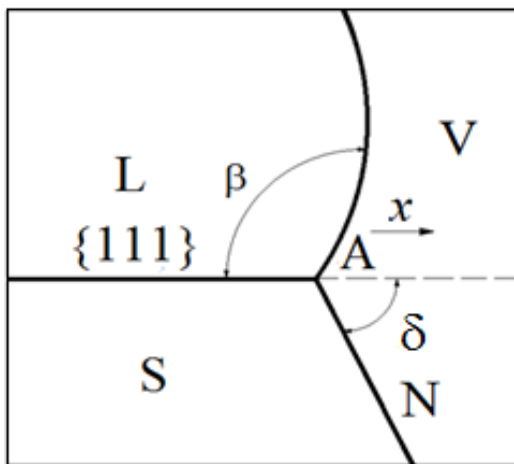
Рис. 24. Остановка контура растекающейся капли у концентрического излома AN (ребра кристалла) на торцевой грани \{111\} ННК [204]
