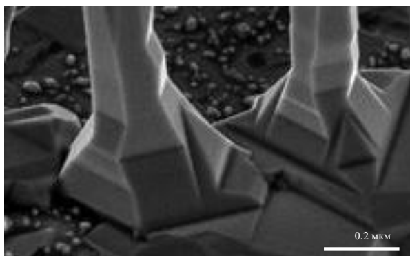
Рис. 36. Огранка боковой поверхности ННК Si, образованная по ПК-механизму
