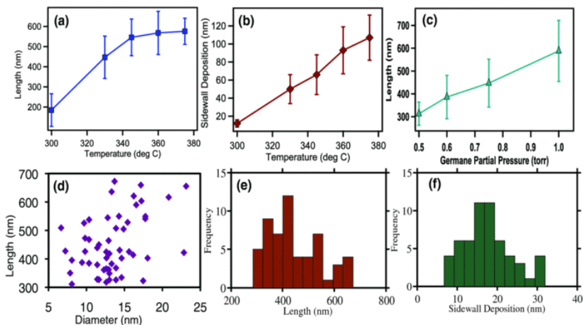
Рис. 14. Температурные зависимости удлинения (а) и толщины осажденного слоя на боковые стенки (б) ННК Ge в процессе роста при парциальном давлении \text{GeH}_4 0,75 Торр; график зависимости длины ННК Ge для разных значений парциального давления германа при 330 °C (с); зависимость длины ННК Ge от диаметра при температуре выращивания T = 330 °C и парциальном давлении германа 0.75 тор (d); гистограммы (е) и (f), показывающие распределение длин ННК и толщин осаждения на боковых гранях для одного и того же образца, соответственно [124]
