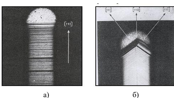
Рис. 28. Протравленное сечение НК Si \{111\} (а) и \{110\} (б), легированного фосфором в процессе изотермического роста с применением жидких капель Au-Si [2]. На фотографиях отчетливо видны примесные полосы
