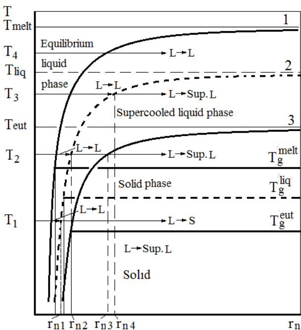
Рис. 22. Диаграмма фазового перехода жидкость→кристалл при нуклеации под каплей двухкомпонентного катализатора в условиях роста ННК [186]
