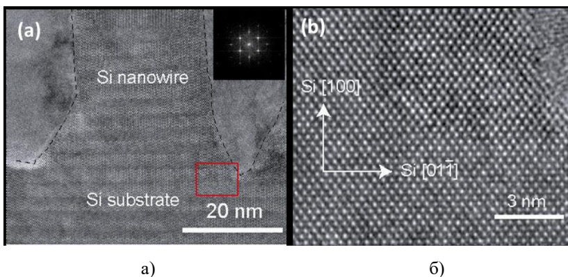
Рис. 3. ПЭМ-изображение ННК Si кристаллографической ориентацией \langle 100 \rangle , выращенного на кремниевой подложке \{100\} темплатным методом, (а) и его увеличенное изображение (б) [61]
