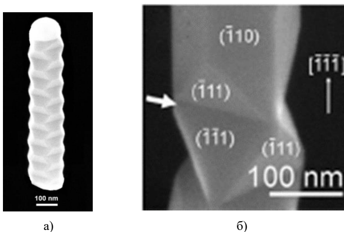
Рис. 35. «Паркетный» полисинтетический двойниковый ННК InAs, выращенный с Au-катализатором методом МOCVD при T=400\text{ }^{\circ}\text{C} , (а) и РЭМ-изображение участка кристалла, содержащего полный октаэдр с пометкой граней семейства \{111\} (б) [244]
