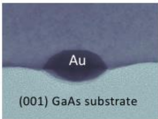
Рис. 11. РЭМ-изображение капли Au-катализатора на подложке (001) GaAs, иллюстрирующее отрицательную кривизну (центр кривизны находится в жидкости) кристалла на границе с равновесной жидкой фазой малого объема [3]
