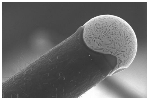
Рис. 23. РЭМ-изображение вершины ННК Si, выращенного в направлении \langle 100 \rangle
