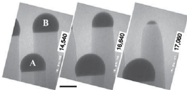
Рис. 9. Покадровые снимки роста ННК Si в сверхвысоковакуумном электронном микроскопе при 928 К. Цифры на снимках показывают время роста в секундах, масштабная линейка – 50 нм [132]
