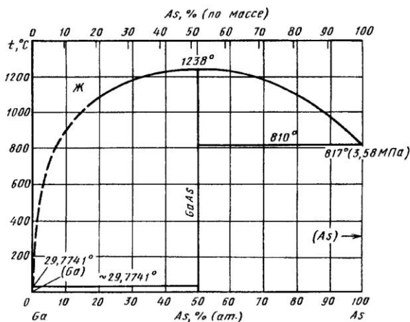
Рис. 34. Диаграмма состояния двухкомпонентной системы Ga–As, образующей химическое соединение GaAs с конгруэнтной точкой плавления [246]
