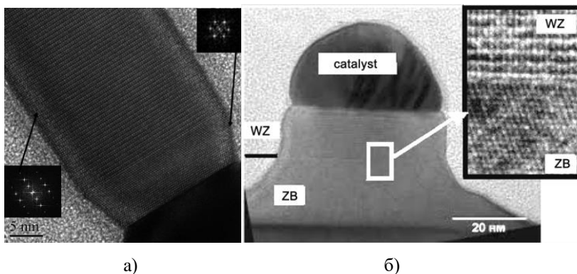
Рис. 29. Переход от вюртцитной структуры (основной кристалл) к кубической (область охлаждения) [3, 65] (а) и трансформация кубической структуры в гексагональную на начальной стадии роста ННК GaAs [3, 65] (б)
