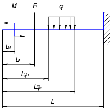
Рис. П1. Схема нагружения инструмента
