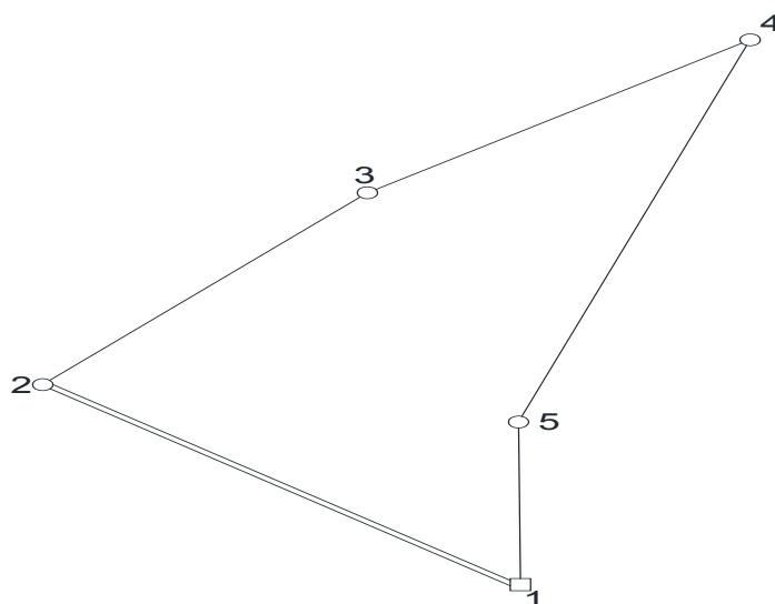
Рис. П.1.Схема теодолитного хода
