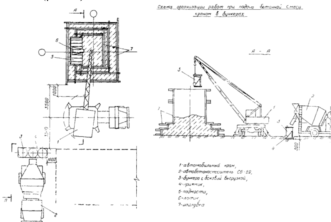
Рис. 15. Возведение монолитных железобетонных фундаментов под колонны
