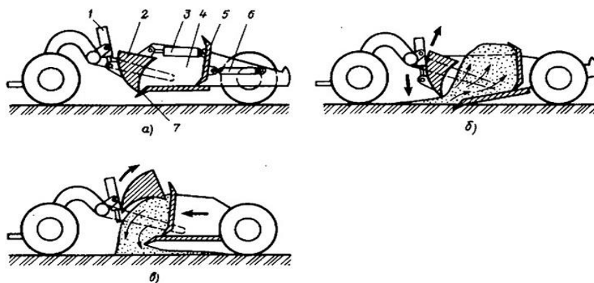
Рис. 8. Схема работы прицепного скрепера:
