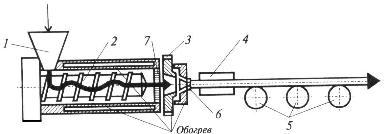
Рис. 11.4. Схема работы экструзионной машины:
