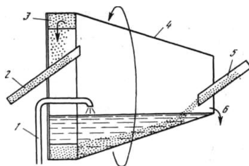
Рис. 3.5. Пескомойка:
