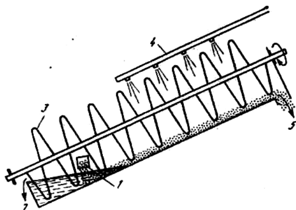
Рис. 3.6. Спиральный классификатор:
