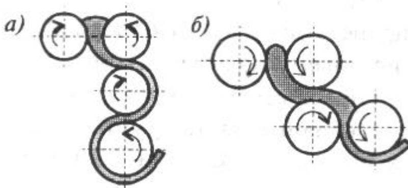
Рис. 11.3. Схема работы четырехвалковых каландров:
