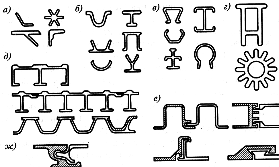
Рис. 15.4. Виды алюминиевых профилей: а) сплошные; б) открытые; в) полуоткрытые; з) замкнутые; д) прессованные панели; е) замковые соединения парных профилей; ж) соединение профилей на защелках
