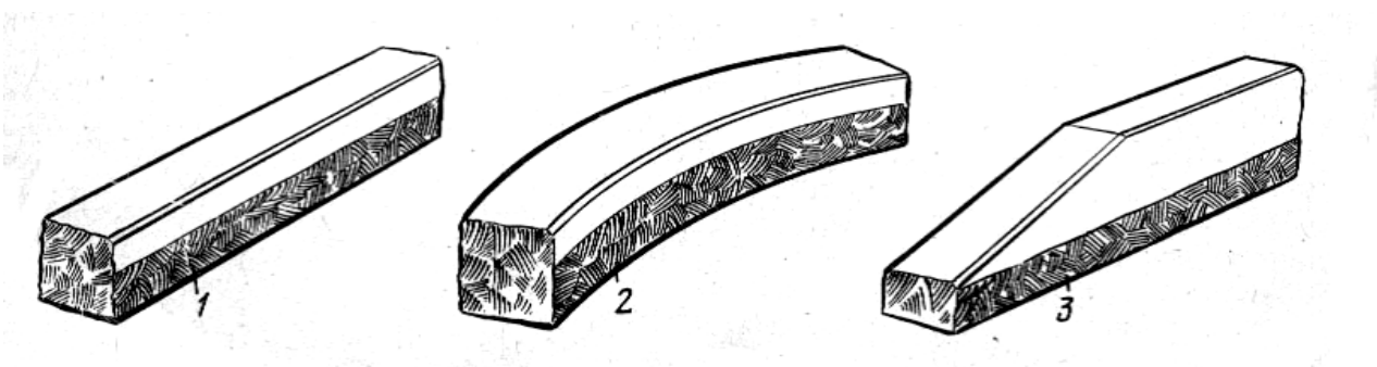
Рис. 3.16. Бортовой камень: 1 – прямой; 2 – лекальный; 3 – для съездов
