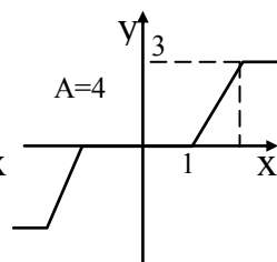
Рис. 3. Ограничение с зоной нечувствительности
