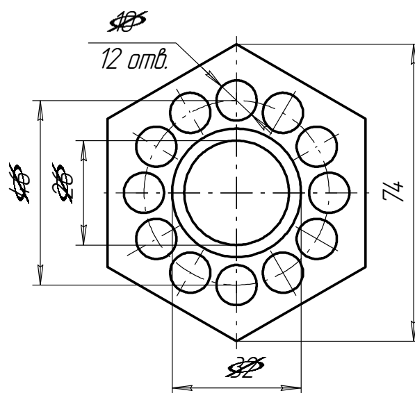
Вариант №4 Крышка
