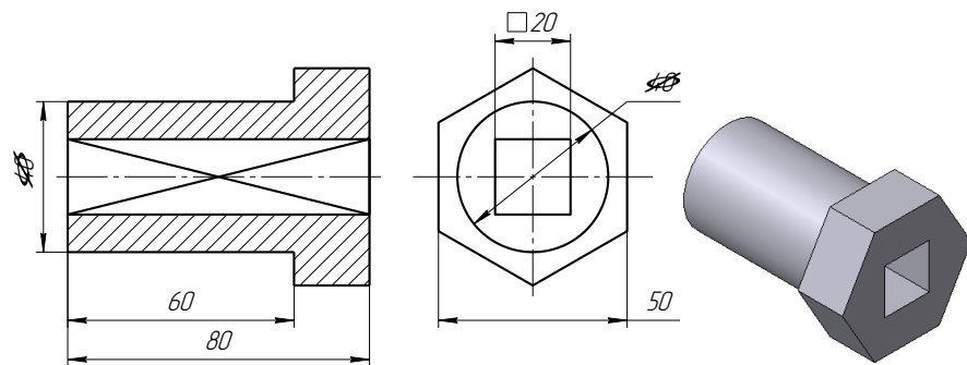
ДСЕ 1
