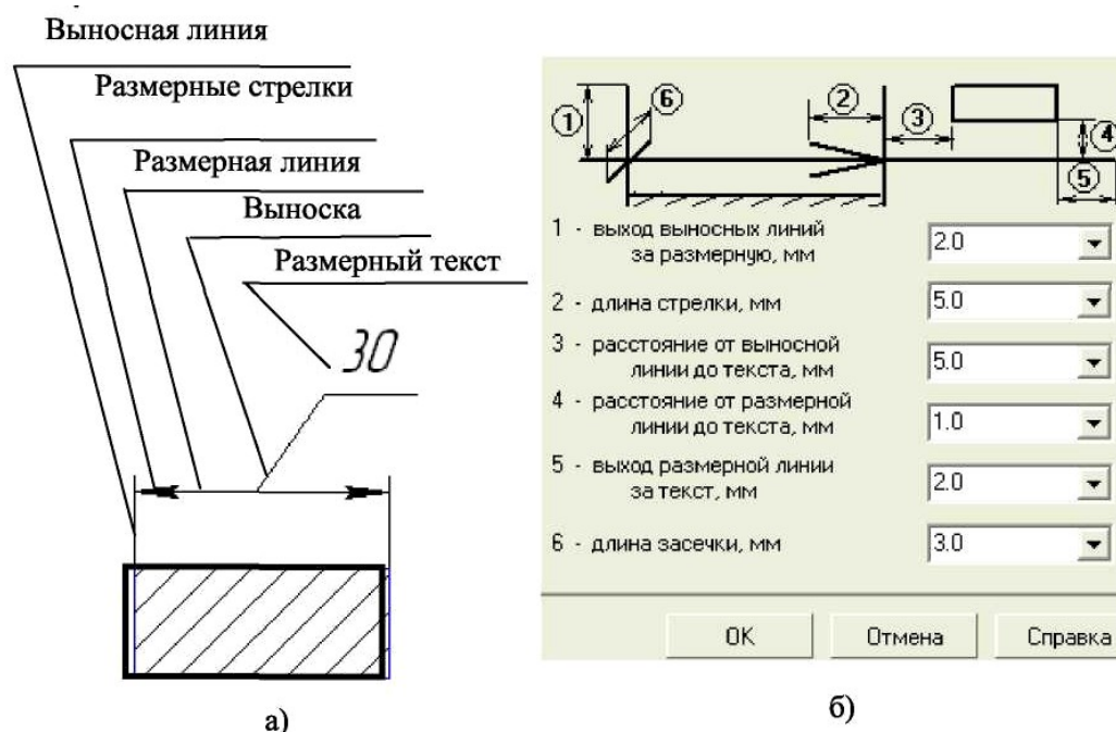
Рис. 2.5. - Параметры отрисовки размеров
