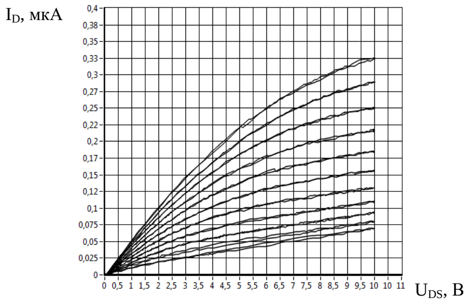
Рисунок Б.2 – ВАХ ТТФТ, измеренная на лабораторном стенде LESO-3
