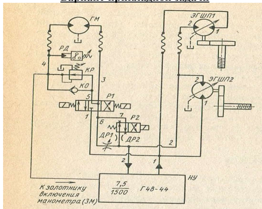
Гидравлическая схема токарного патронного станка с ЧПУ мод. 16K20РФ3
