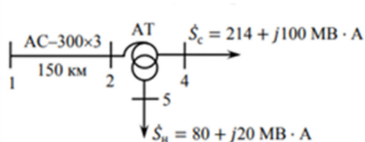
Рис.1 Схема сети
