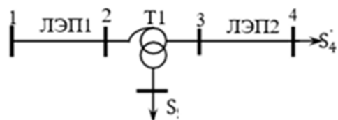
Рис.1. Исходная схема сети
