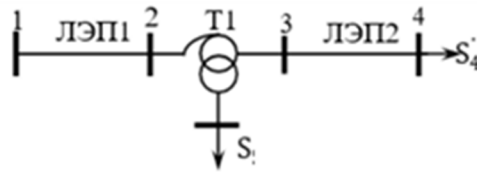
Рис.1. Исходная схема сети
