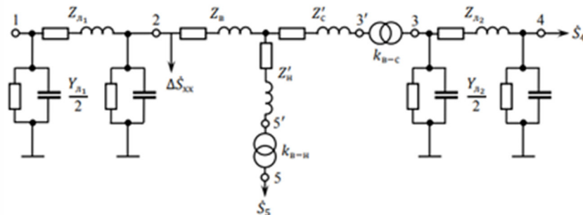
Рис. 2. Схема замещения сети
