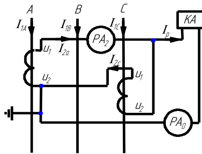
Рис.1. Схема соединения трансформаторов тока и обмоток токового реле по двухфазной однорелейной схеме.
