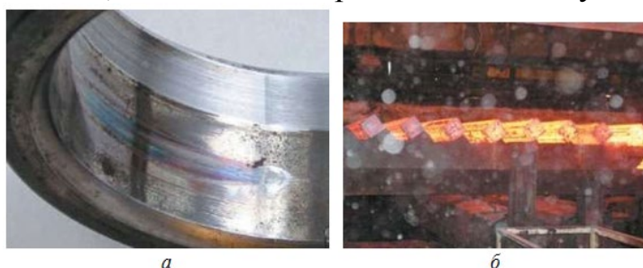
Рис. 11.4. Цвета побежалости и цвета каления а) цвета побежалости на посадочной поверхности внутреннего кольца подшипника при схватывании и провороте; б) изменение цветов каления при охлаждении непрерывно литой заготовки на холодильнике МНЛЗ
