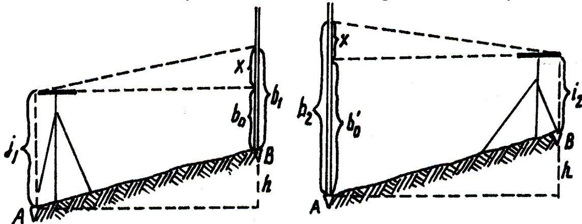
Рис. 7.3. Поверки оси цилиндрического уровня двойным нивелированием
