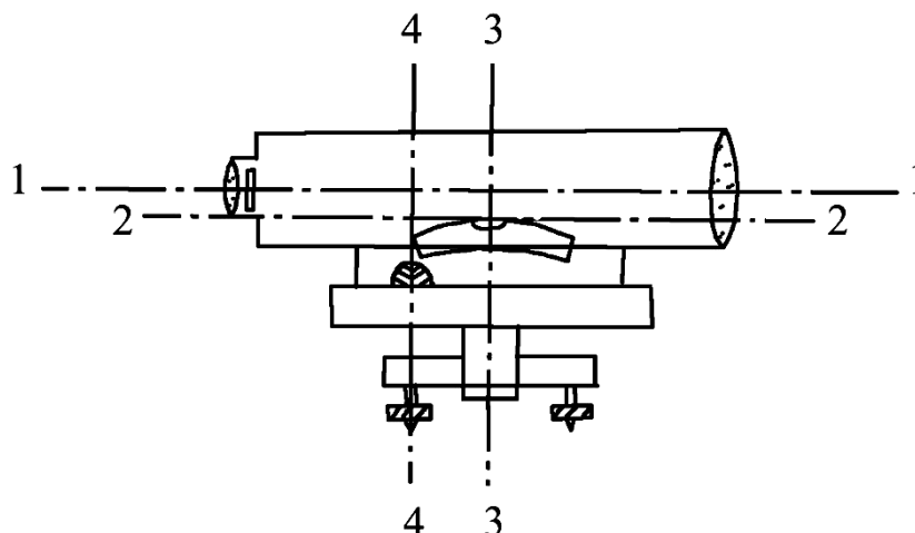
Рис. 7.1. Схема осей нивелира:
