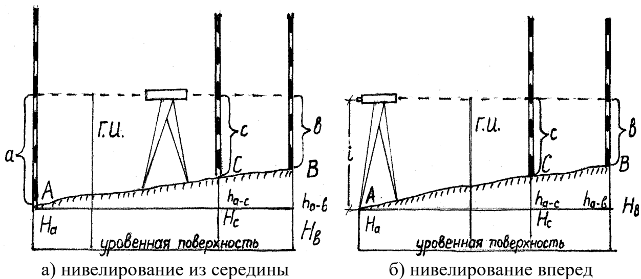
Рис. 5.6. Схемы геометрического нивелирования h_{a-b} = a - b ; h_{a-b} = i - b
