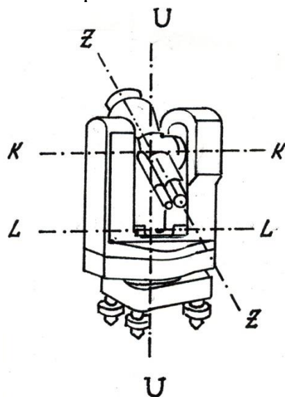
Рис. 3.1. Оси теодолита
