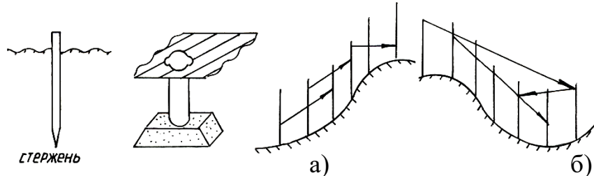
Рис. 1.1. Закрепление линий
