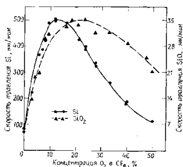
Рис. 1.11. Влияние добавок в плазму O_2 в плазму CF_4
