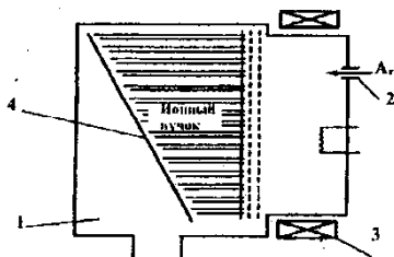
Рис. 1.2. Схема установки ионно-лучевого травления:
