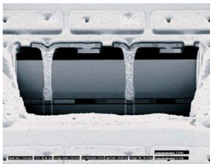
Рис. 2.6. Сквозные отверстия в кремнии
