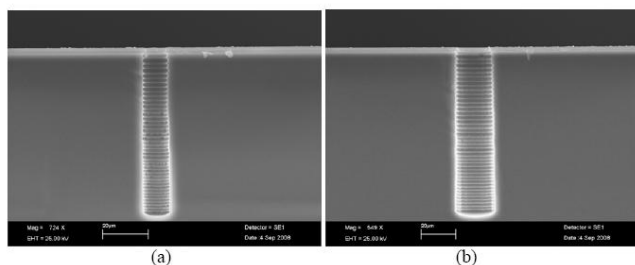
Рис. 1.16. Отверстие диаметром 10 мкм, протравленное на глубину 72 мкм при скорости травления 14,3 мкм/мин (а). Отверстие диаметром 20 мкм, протравленное на глубине 96 мкм при скорости травления 19.0 мкм/мин (б)
