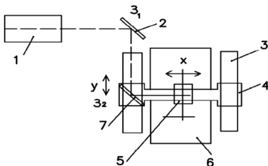
Рис. 2.2. Схема портальной установки для лазерного раскроя листа: 1 -СО лазер; 2 - неподвижное зеркало Z_1 ; 3 - направляющие портала; 4 - портал, перемещающийся по направляющим (ось Y); 5 - каретка с зеркалом Z_2 и оптическим резаком, перемещающаяся по portalу (ось X); 6 - неподвижный стол для размерной обработки детали; 7 - подвижное зеркало Z_2 , укрепленное на портале
