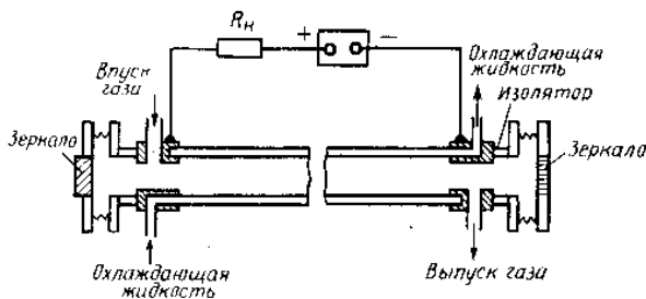
Рис. 2.9. Устройство \text{CO}_2 -лазера с продольной прокачкой газа
