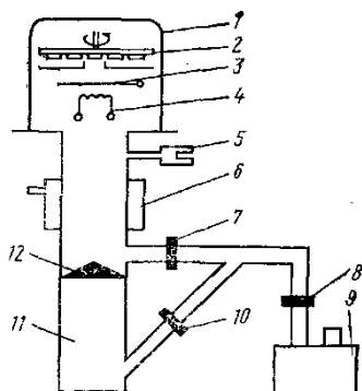
Рис. 3.3. Схема установки термовакuumного испарения
