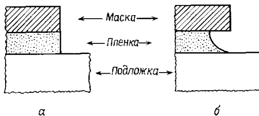
Рис. 1.7. Идеальные профили травления для а - полностью анизотропного ( A = 1 ) и б - изотропного ( A = 0 ) травления при отсутствии подтравки маски
