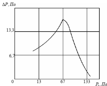
Рис. 1.10. Прирост давления \Delta P в реакторе
