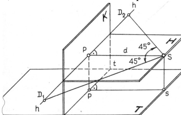
Рис. 7. Элементы перспективы
