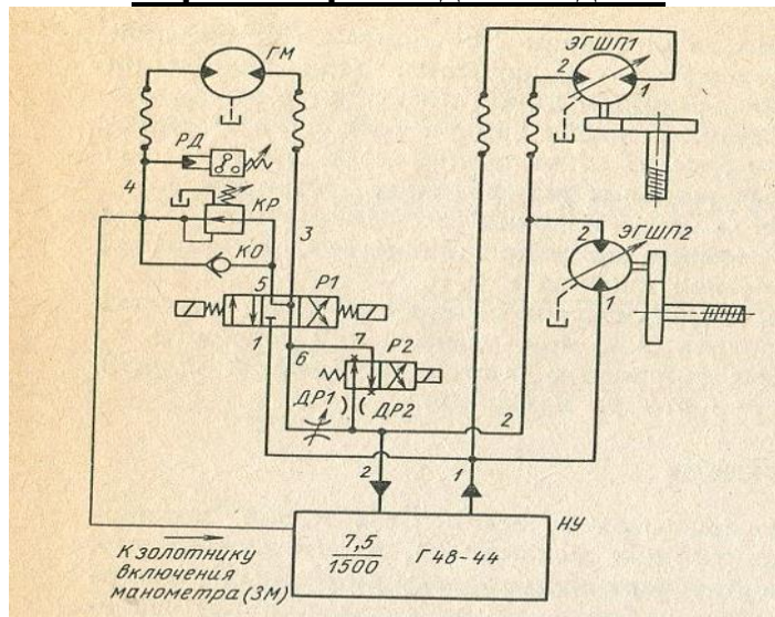
Гидравлическая схема токарного патронного станка с ЧПУ мод. 16К20РФ3
