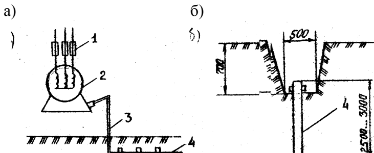
Рис. 6. Устройство заземлителя: а – схема заземляющей сети; б – расположение одиночного заземлителя; 1 – плавкие вставки; 2 – электродвигатель; 3 – соединительная полоса; 4 – трубчатый заземлитель
