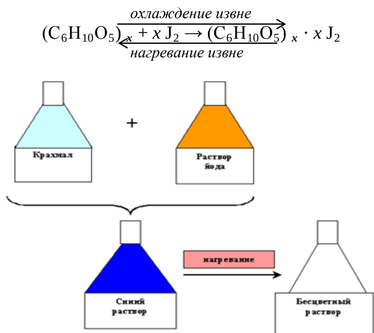
Рис.10 Смещение равновесия
