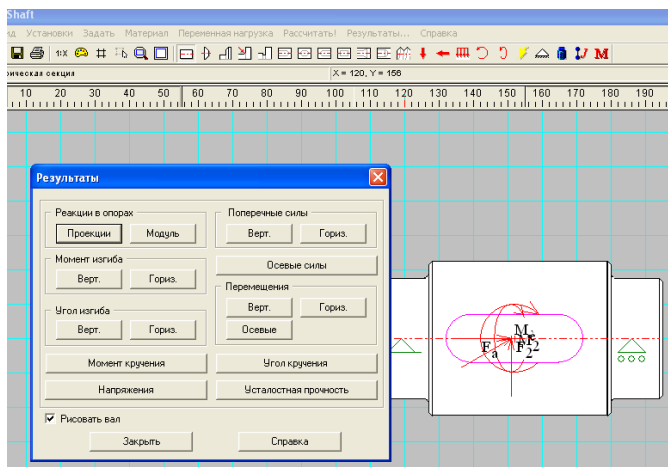
Рис. 4.15. Вывод результатов расчета
