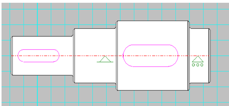
Рис.4.7. Вал с опорами и шпоночными пазы
