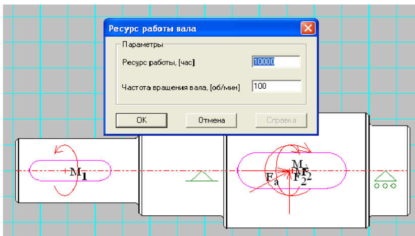
Рис. 4.14. Ввод дополнительных данных для общего расчета
