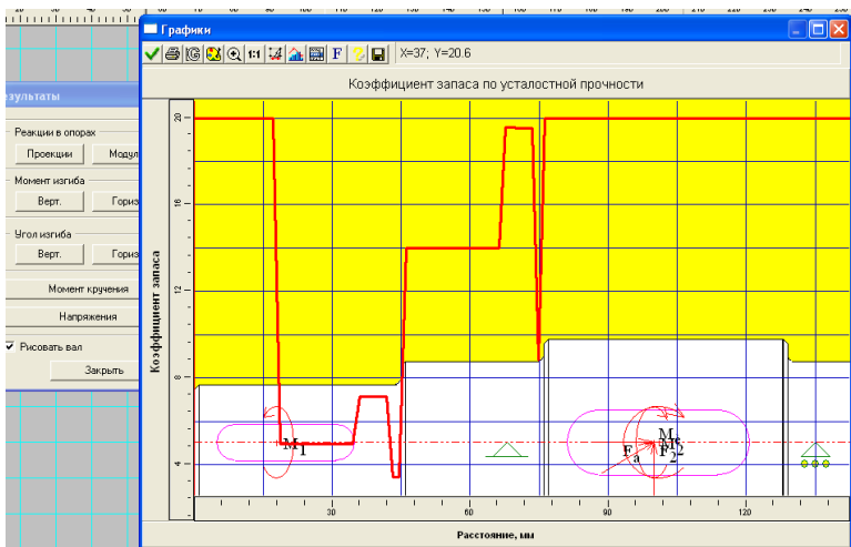
Рис. 4.16. Результаты усталостного расчета вала
