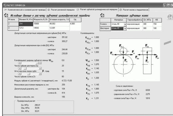
Рис. 1.4. Диалоговое окно для предварительного расчета зубчатой передачи
