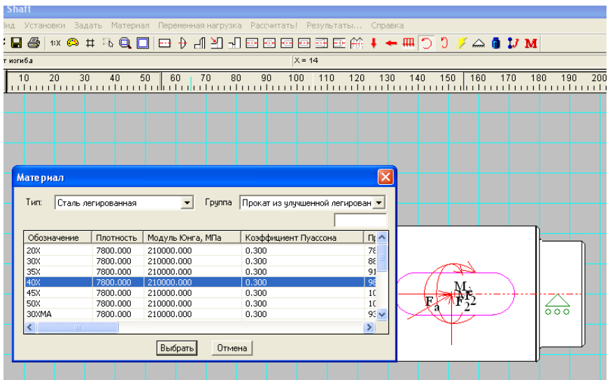
Рис. 4.13. Выбор материала вала
