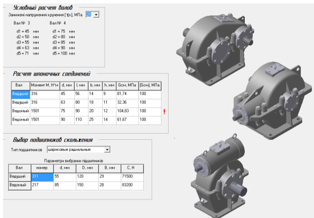
Рис. 1.5. Диалоговое окно для предварительного расчета валов, шпонок и подшипников
