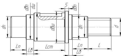
Рис. 3.1. Конструктивно проработанная схема вала
