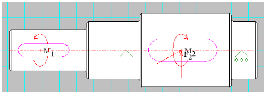
Рис. 4.10. Нанесение усилий окружного, радиального и крутящего момента
