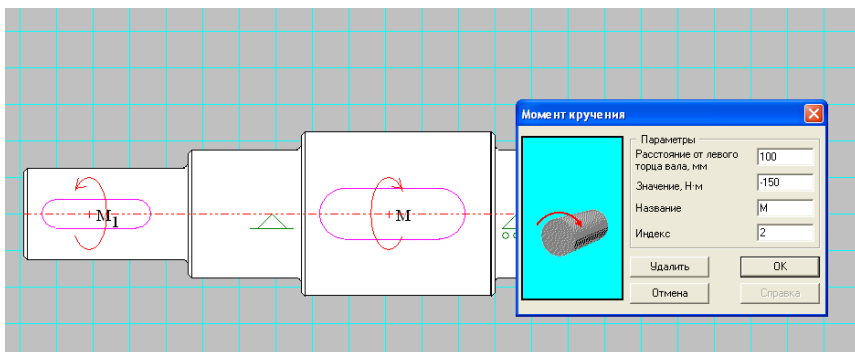
Рис. 4.8. Действие крутящего момента
