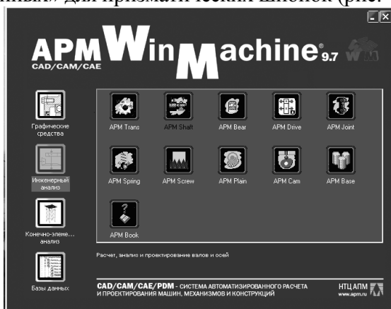
Рис. 4.1. Запуск программы
