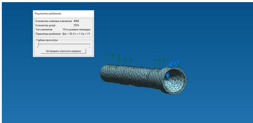
Рисунок 5.5. Конечно-элементная модель вала
