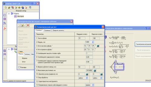
Рис. 2.3. Заполнение таблицы расчетными данными
