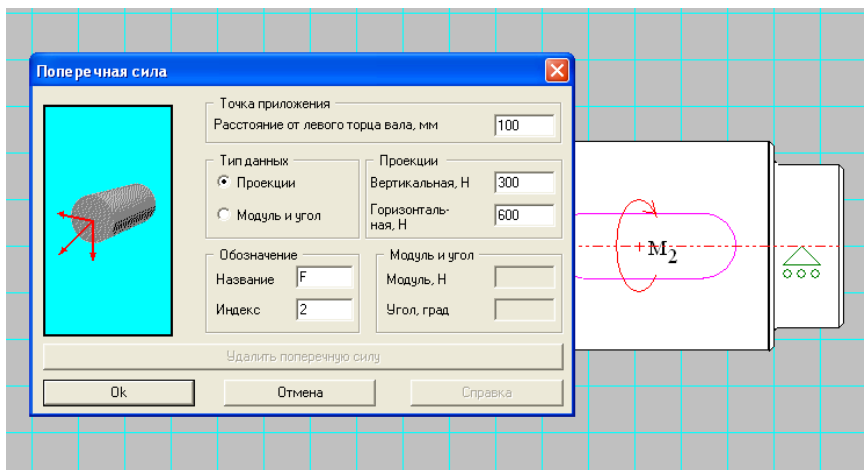
Рис. 4.9. Нанесение усилий окружного и радиального
