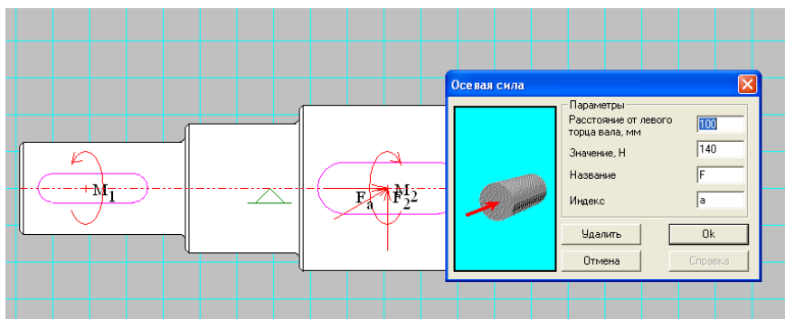
Рис. 4.11. Нанесение осевого усилия
