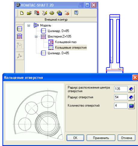
Рис. 2.10. Параметры кольцевых отверстий
