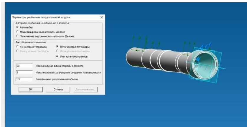
Рисунок 5.4. Разбиение вала на конечные элементы
