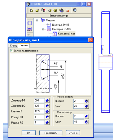
Рис. 2.8. Формирование параметров кольцевых пазов
