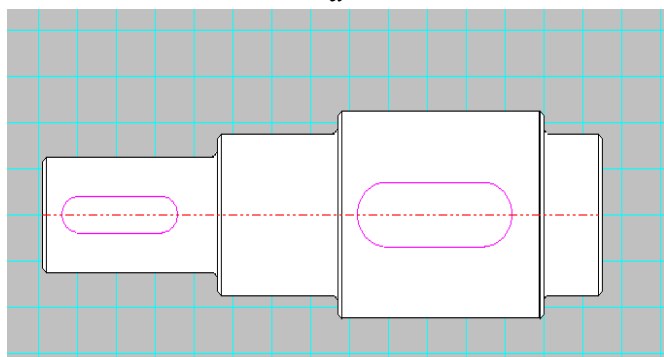
Рис. 4.5. Нанесение шпоночных пазов
