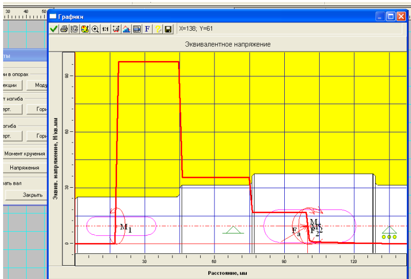
Рис. 4.17. Эквивалентные напряжения вала
