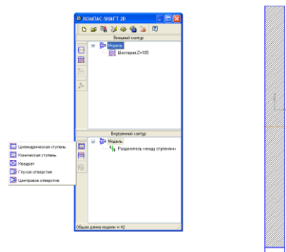
Рис. 2.5. Формирование отверстия для вала
