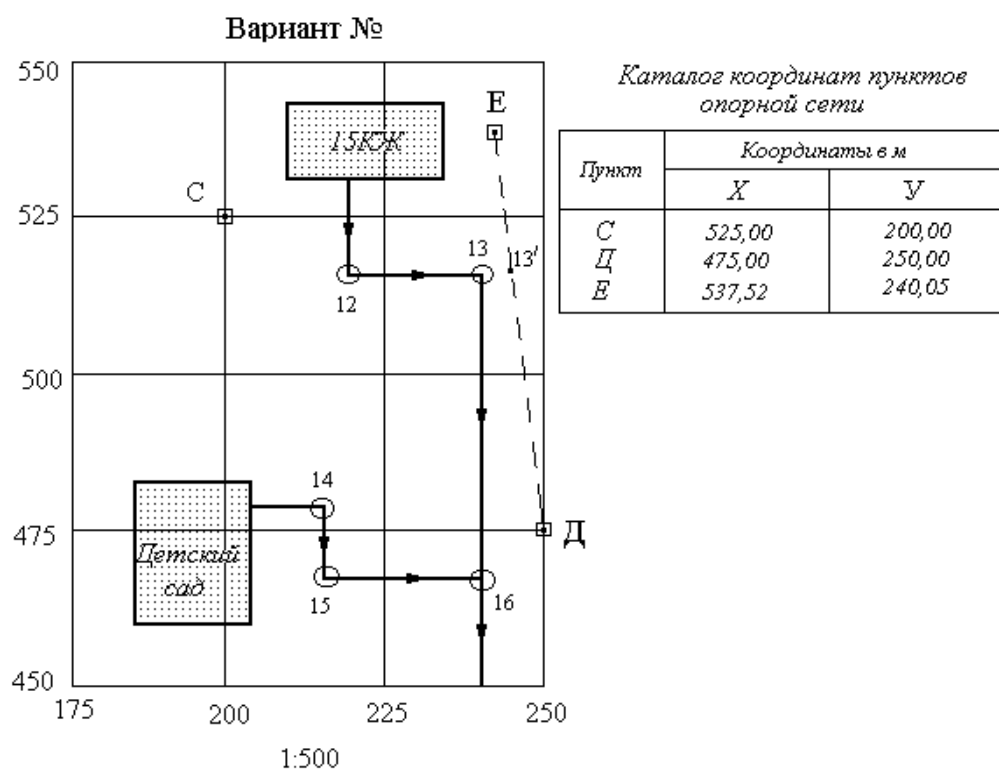
Рис. 3. Схема расположения колодцев подземных коммуникаций
