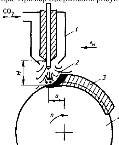
Рисунок 1 - Схема наплавки в среде углекислого газа (1- наплавочная головка; 2 - зона подачи CO 2 ; 3 - наплавленный металл; 4 - деталь)
