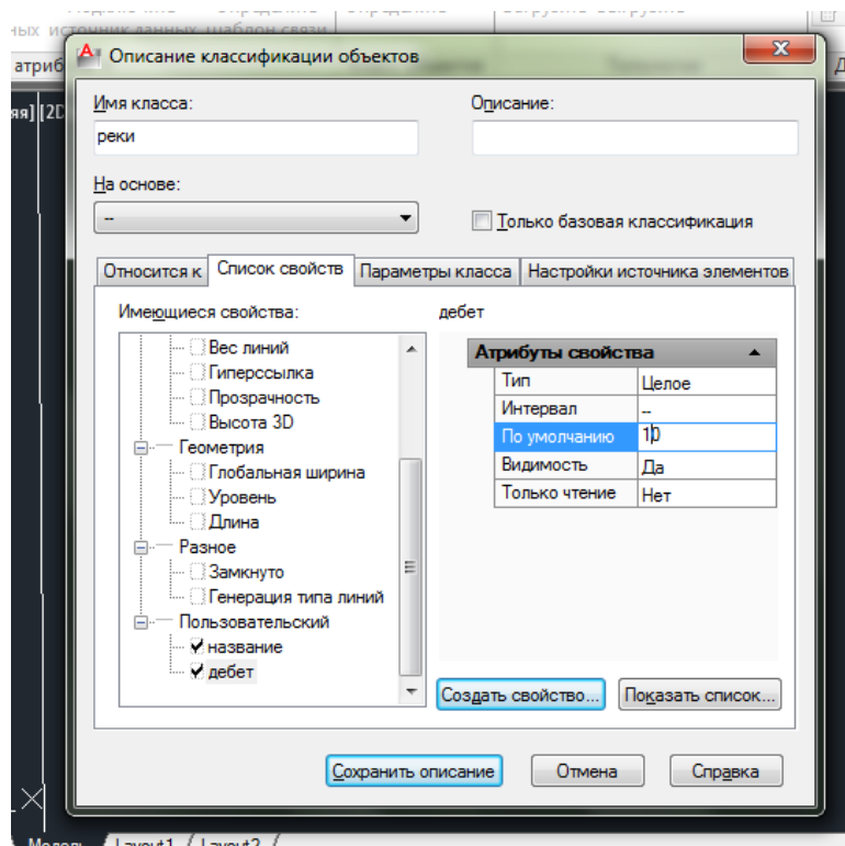
Рис.7. Создание свойств
