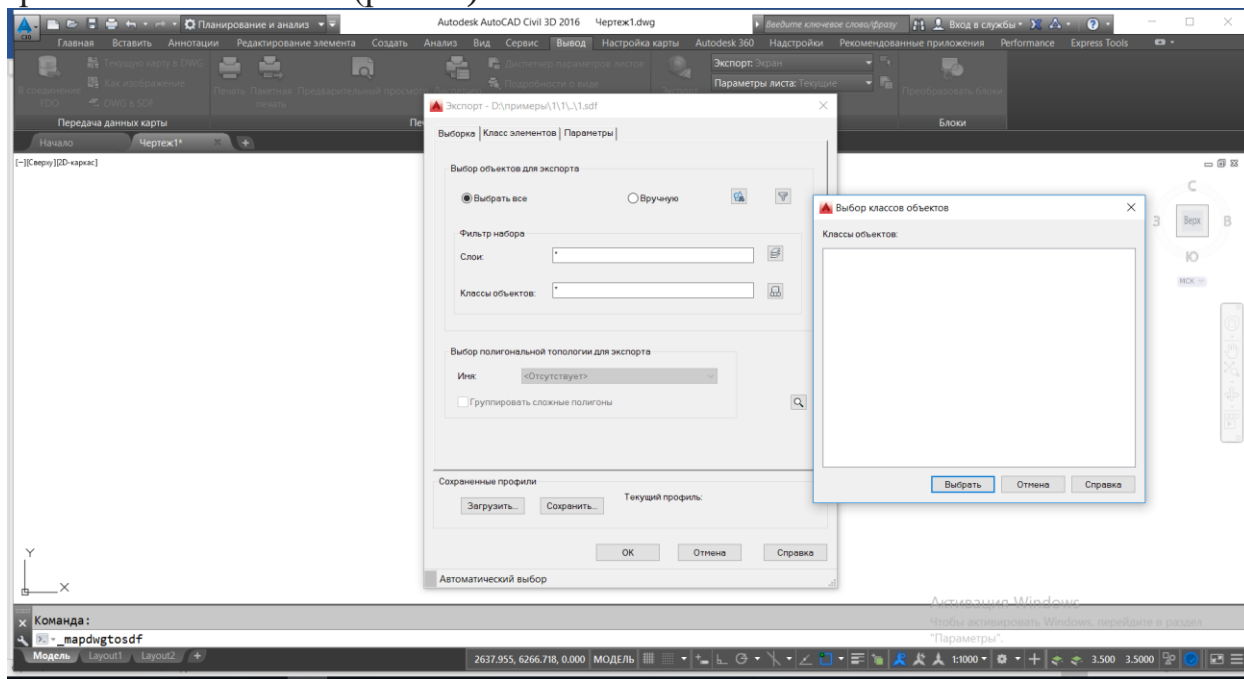
Рис.12. Экспорт данных
