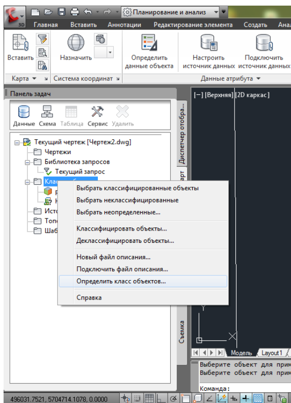
Рис.8. Классификация объектов
