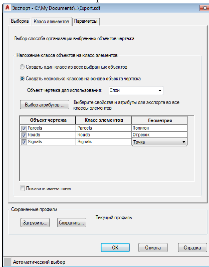
Рис.12. Экспорт данных
