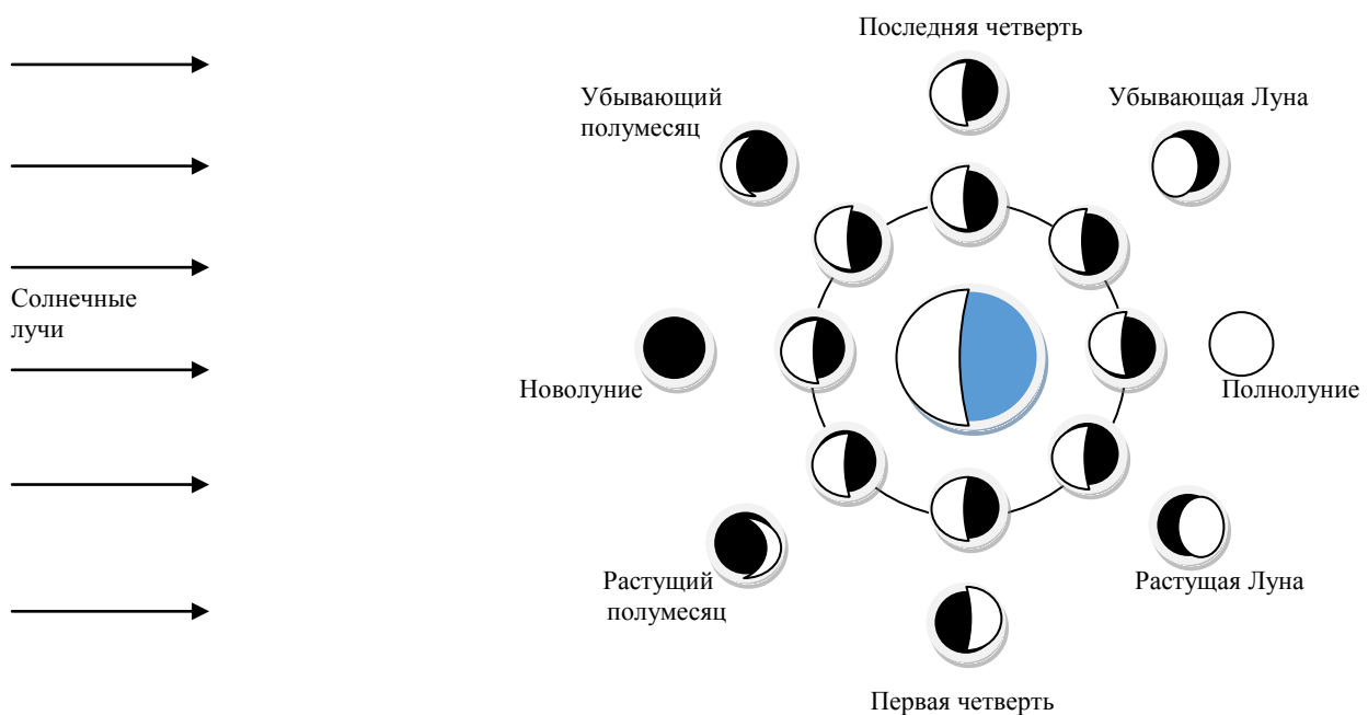
Рис. 6. Фазы Луны
