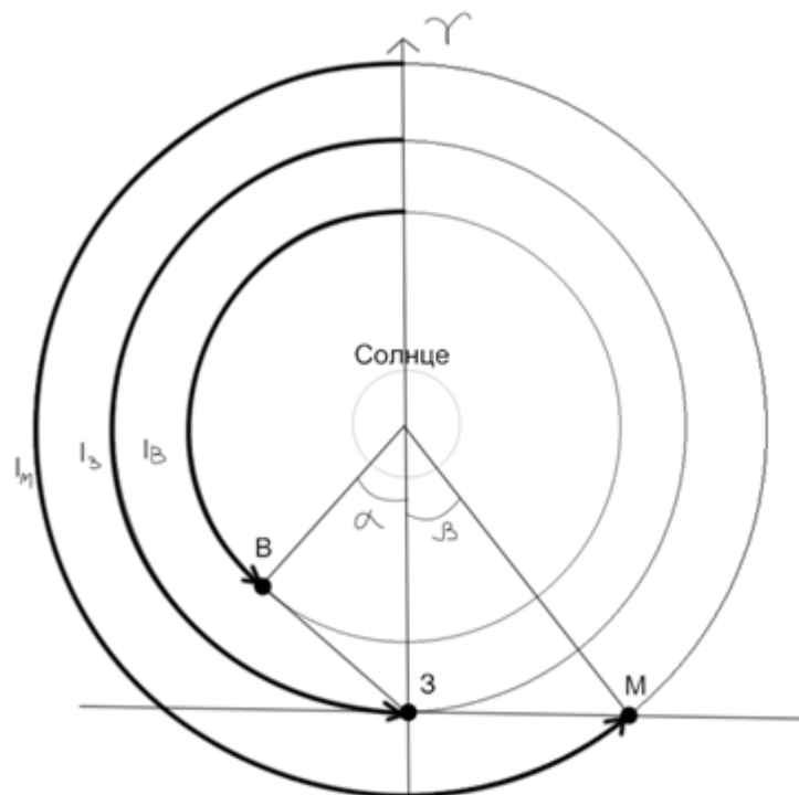
Рис. 5. Конфигурации планет
