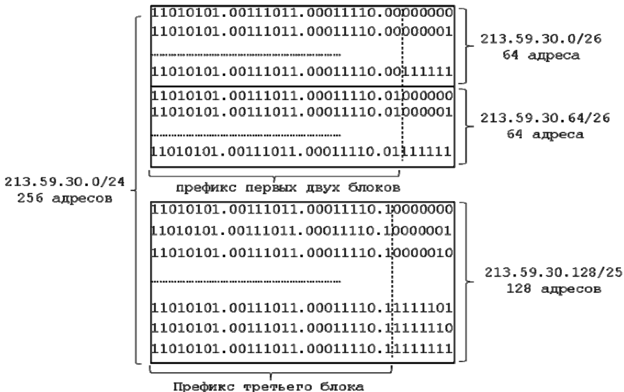
Рис. 10. Распределение адресов
