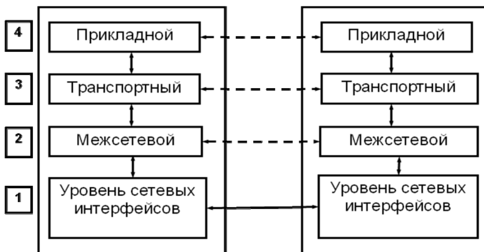
Рис. 1. Структура стека TCP/IP
