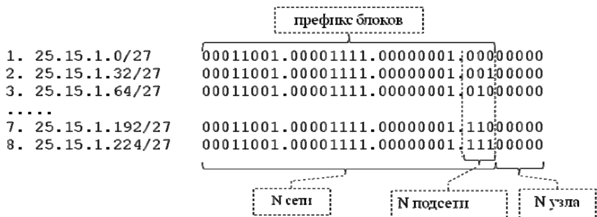
Рис. 19. Варианты номеров сетей
