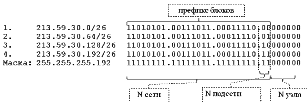
Рис. 8. Номера сетей
