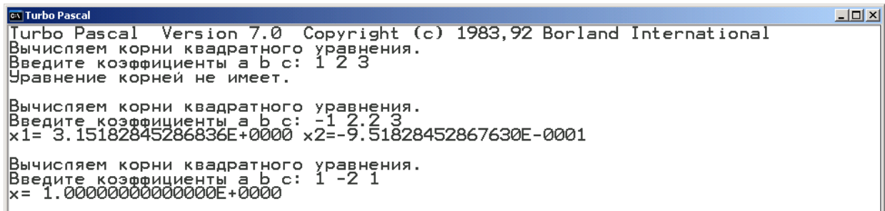
Рис.1. Программная реализация разветвляющегося алгоритма с использованием оператора if
