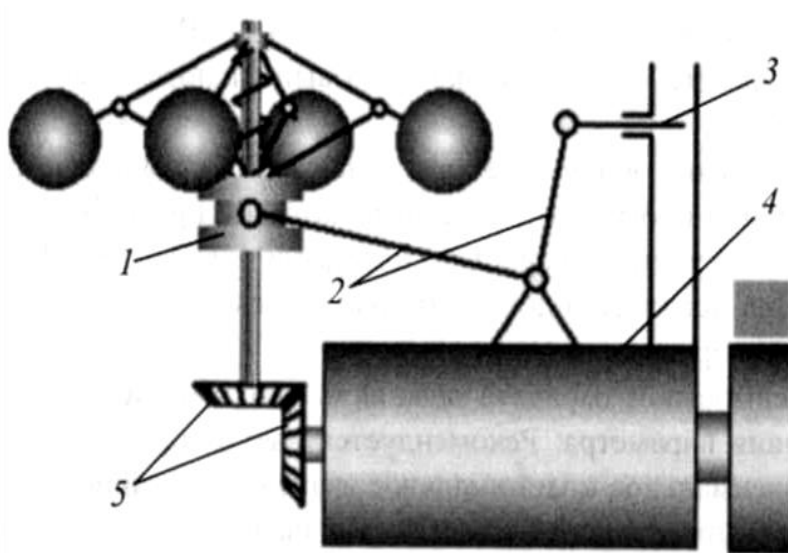
Рис. 1. Схема САУ скоростью вращения двигателя
