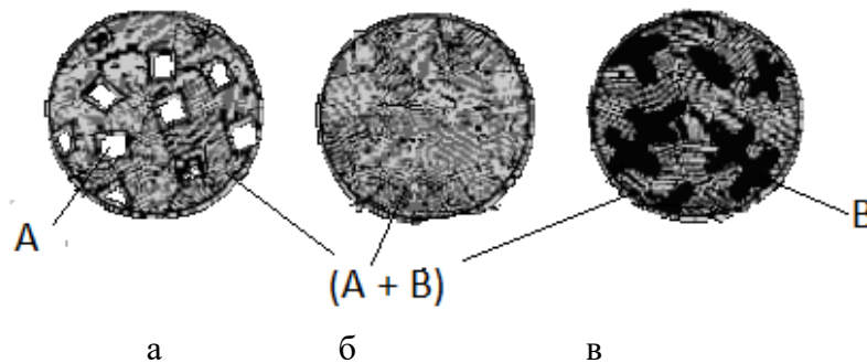
Рис. 9. Схема микроструктур сплавов, образующих механические смеси чистых компонентов: а – доэвтектического, б – эвтектического, в – заэвтектического
