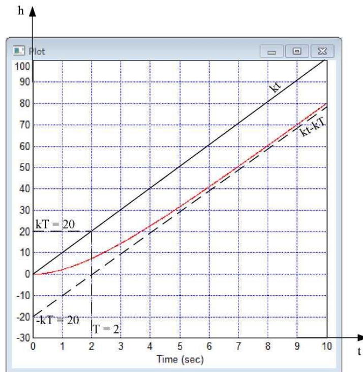
Рис. 4. Переходная функция интегрирующего звена с k=10 и T=2 сек
