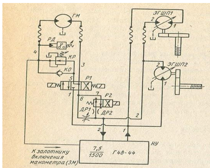
Гидравлическая схема токарного патронного станка с ЧПУ мод. 16K20PФ3
