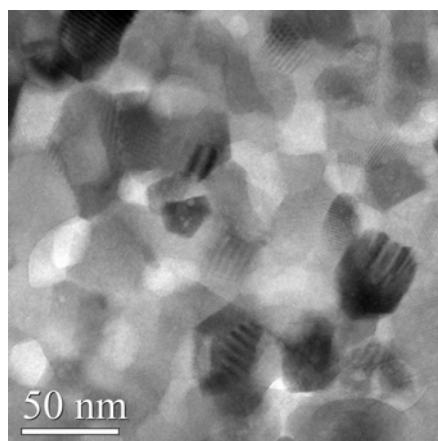
Рис. 2 Светлопольное ПЭМ-изображение нанокристаллической керамики
