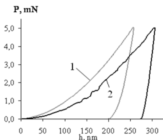
Рис. 6 Диаграммы P-h поверхности со стороны межфазной границы и свободной поверхности твердого раствора на основа Mo-Cu, полученные методом наноиндентирования
