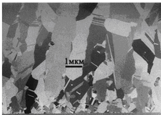
Рис. 5 ПЭМ-изображение поперечного среза фольги на основе твердого раствора Mo-Cu, полученной методом вакуумного осаждения
