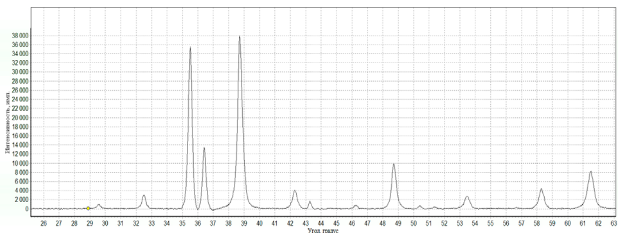
Рис. 4 Рентгеновская дифрактограмма нанокристаллических порошков, включающих Си и О
