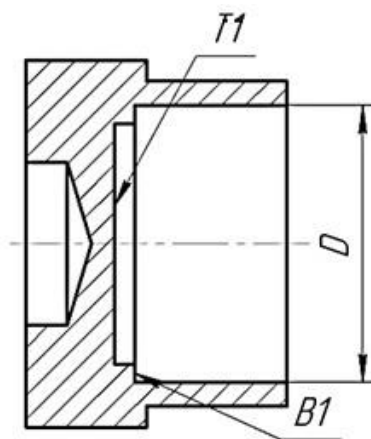
Рис. 4. Заглушка
