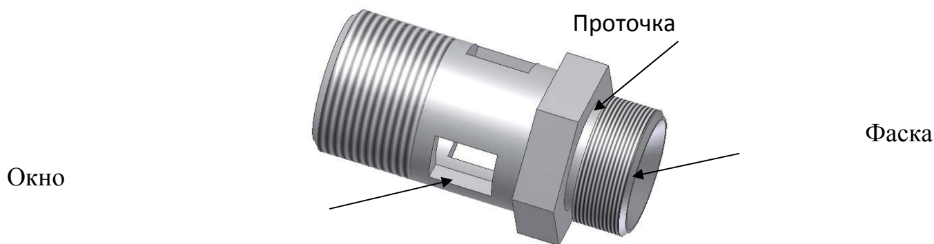
Рис. 2.1. Модель втулки
