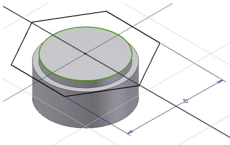
Рис. 2.15. Эскиз шестиугольника
