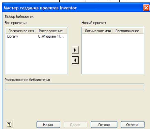
Рис. 1.5. Выбор библиотек
