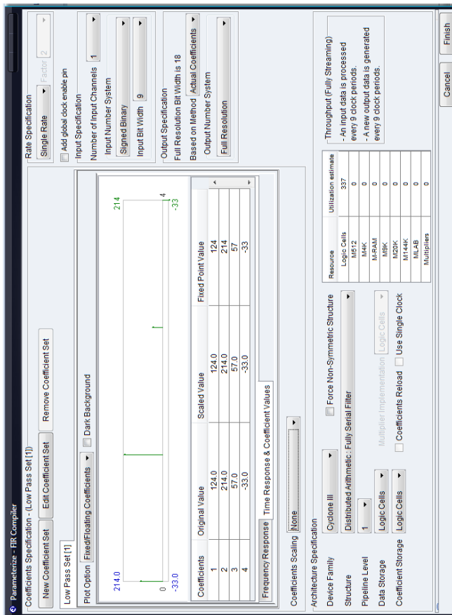
Рис. 6.27. Настройки мегафункции Altera fir_compiler_v13_1. Показана импульсная характеристика КИХ-фильтра (коэффициенты загружаются целочисленными, предварительно умноженные на масштабный множитель 256)
