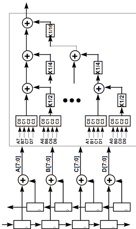
Рис. 2.19. Использование параллельного векторного умножителя четырех 8-разрядных сигналов на четыре 8-разрядные константы в составе КИХ-фильтра на восемь отводов с симметричными коэффициентами в базисе ПЛИС XC4000, построенного с использованием параллельной распределенной арифметики
