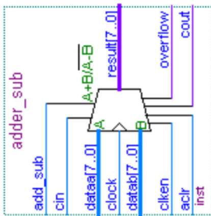
Рис. 2.39. Сумматор/вычитатель на базе мегафункции LPM_ADD_SUB
