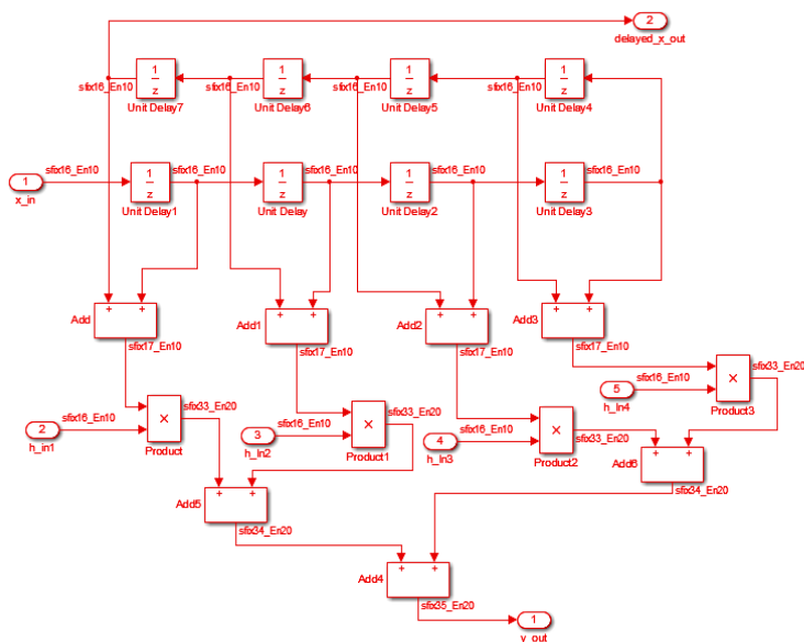
Рис. 2.6. Имитационная модель симметричного КИХ-фильтра на восемь отводов с указанием формата сигналов. Нижний уровень иерархии. Структура фильтра в элементах системы Matlab/Simulink
