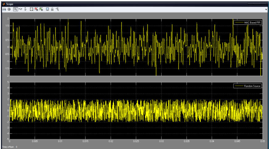
Рис. 5.25. Имитационное моделирование в системе Matlab/Simulink КИХ-фильтра на 34 отвода с использованием одного МАС-блока и блочной памяти
