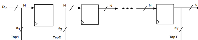
Рис. 3.26. Линия задержки КИХ-фильтра на регистрах
