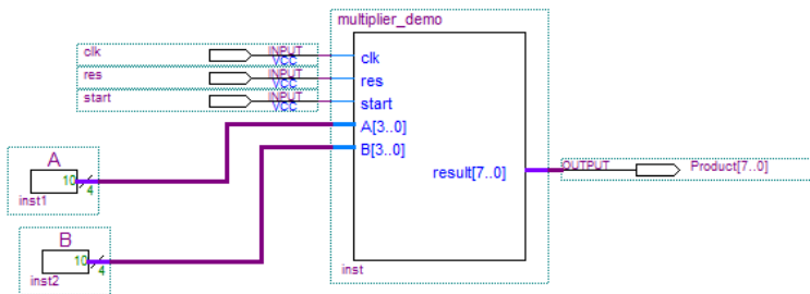
Рис. 1.34. Умножитель размерностью 4х4. Верхний уровень иерархии схемы
