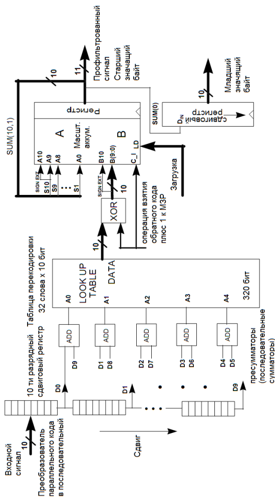
Рис. 2.21. Симметричный КИХ-фильтр со структурой десять отводов десяти бит с использованием последовательной распределенной арифметики
