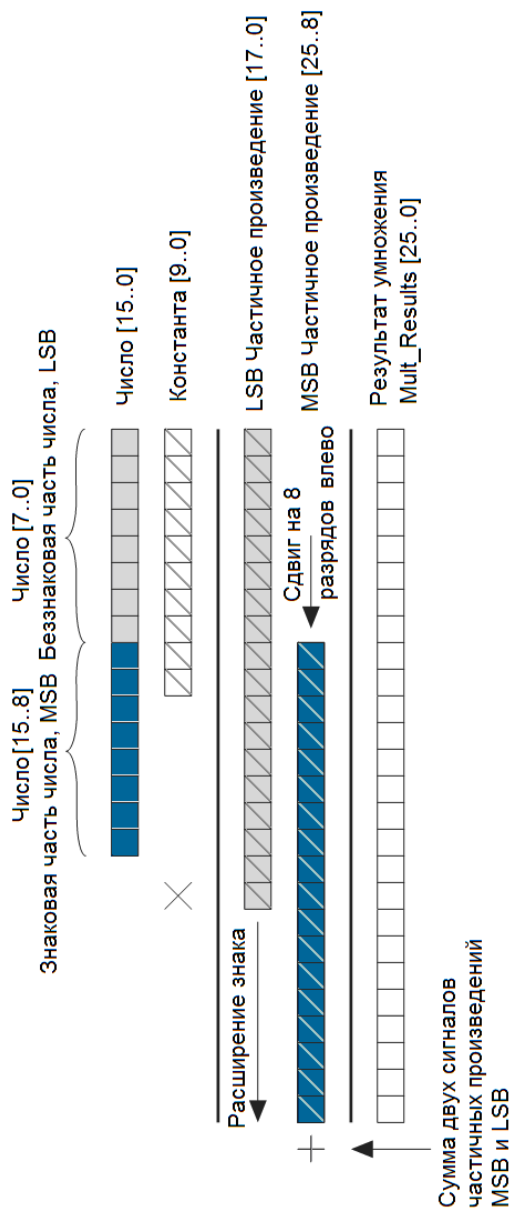
Рис. 1.30. Идея параллельного умножения 16-разрядного числа на 10-разрядную константу
