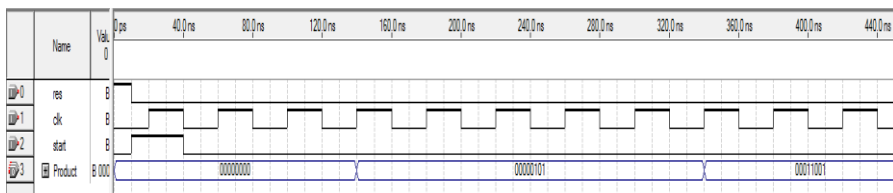
Рис. 1.39. Тестирование умножителя на примере умножения 5х5. Результат 25
