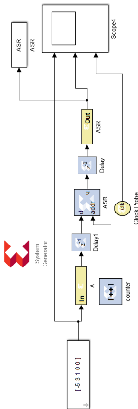
Рис. 5.38. Исследование латентности ASR-блока при подключении задержки на один такт на его вход и задержки на два такта на выход
