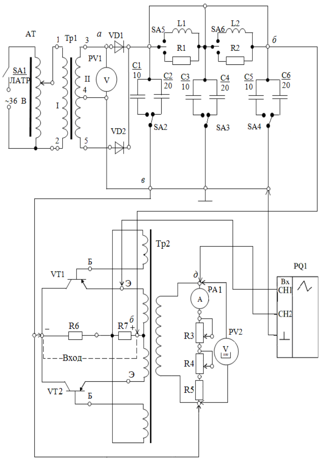
Схема лабораторной установки для проведения измерений параметров а) параметрического стабилизатора напряжения б) компенсационного стабилизатора напряжения в) транзисторного инвертора напряжения
