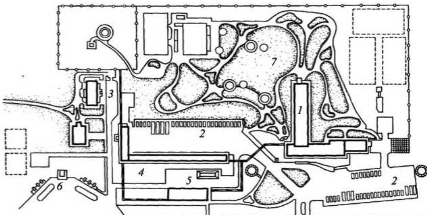
Рис.10. Архитектурно-планировочная организация участка мотеля: 1 – здание мотеля с помещениями общественного питания, администрации; 2 – автостоянка; 3 – хозяйственное сооружение; 4 – гараж; 5 – сооружение тех- нического обслуживания автомобилей; 6 – сквер; 7 - зона отдыха
