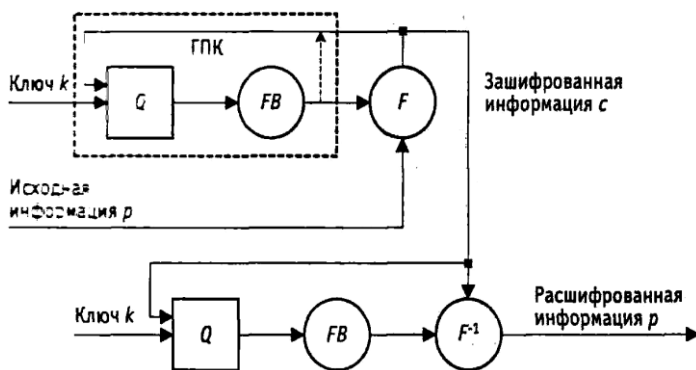
Рис. 2 - Шифрование информации методом гаммирования с обратной связью (схема самосинхронизирующегося поточного шифра): G – генератор псевдослучайных кодов, Q – элементы памяти ГПК, FB – функция обратной связи ГПК, F – линейная или нелинейная функция, F^{-1} – функция, обратная F
