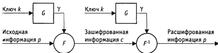
Рис.1 - Шифрование информации методом гаммирования (схема синхронного поточного шифра): G – генератор псевдослучайных кодов, F – линейная или нелинейная функция гаммирования, F^{-1} – функция, обратная F , \gamma - гамма шифра
