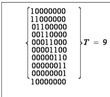
Рис. 4 - Последовательность генерируемых ключей для 8-ми разрядного скремблера
